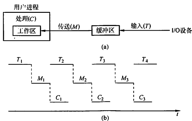
图 5.6 单缓冲工作示意图
