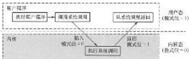
图 1.3 系统调用执行过程
