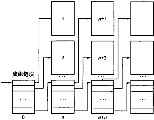
图 4.21 成组链接法示意图
