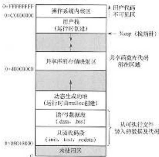
图 3.3 内存中的一个进程
