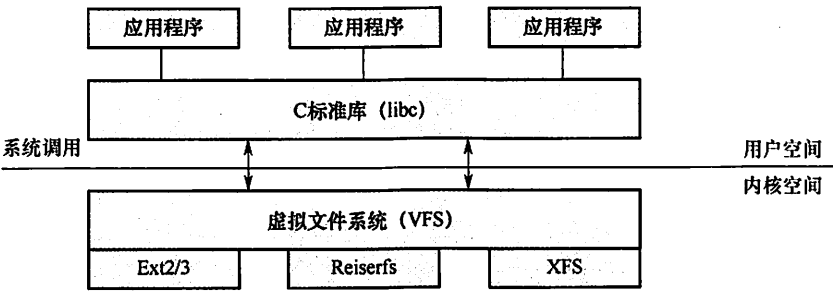
图 4.22 虚拟文件系统的示意图
