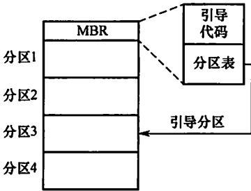
图 5.15 Windows 磁盘的引导
