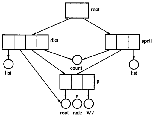
图 4.14 无环图目录结构
