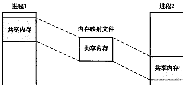
图 3.28 采用内存映射 I/O 的共享内存
