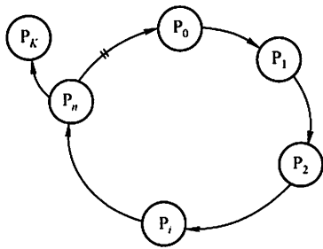
图 2.14 满足条件但无死锁
