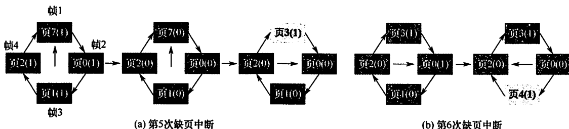
图 3.27 缺页中断时替换指针扫描示意图
