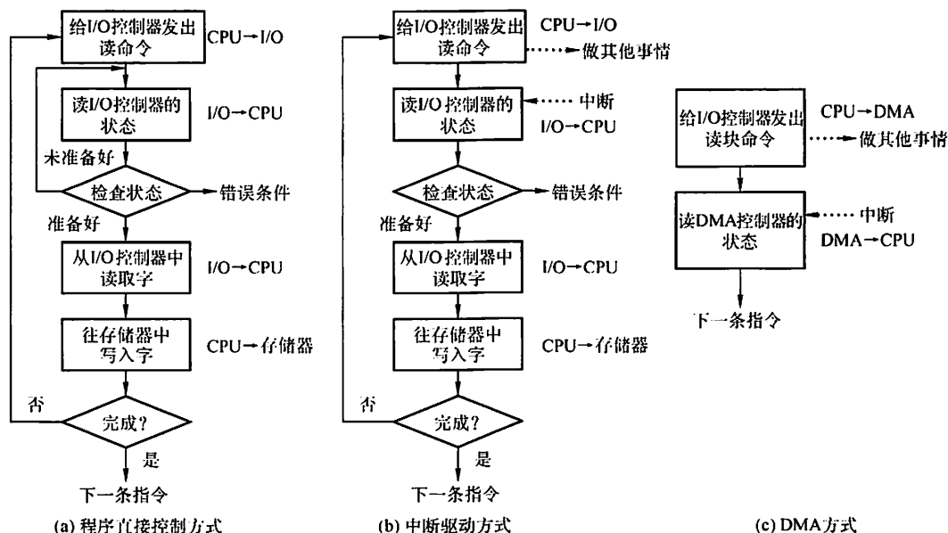
图 5.3 I/O 控制方式
