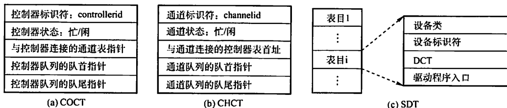
图 5.11 控制器控制表 COCT、通道控制表 CHCT 和系统设备表 SDT
