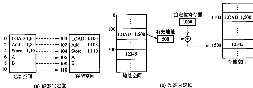
图 3.2 重定位类型
