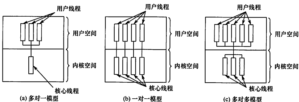
图 2.6 多线程模型
