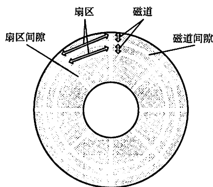
图 5.13 磁盘盘片
