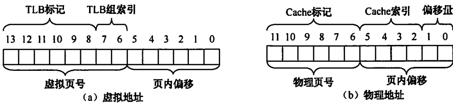
图 3.29 地址结构
