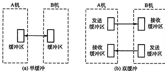
图 5.8 双机通信时缓冲区的设置
