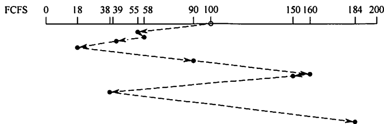
图 5.16 FCFS 磁盘调度算法
