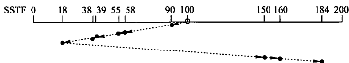
图 5.17 SSTF 磁盘调度算法
