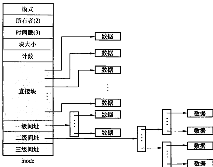
图 4.10 UNIX 系统的 inode 结构示意图
