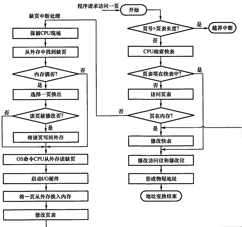
图 3.21 请求分页中的地址变换过程
