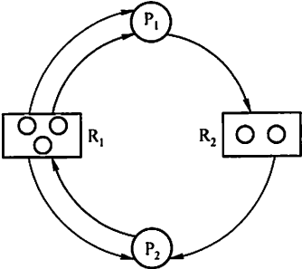
图 2.15 资源分配示例
