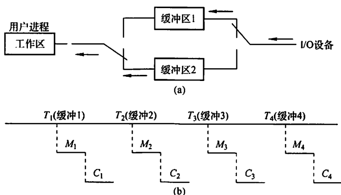
图 5.7 双缓冲工作示意图
