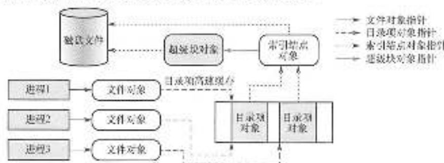
图 4.24 进程与 VFS 对象之间的交互
