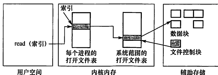
图 4.3 内存中文件的系统结构
