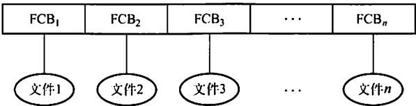
图 4.11 单级目录结构
