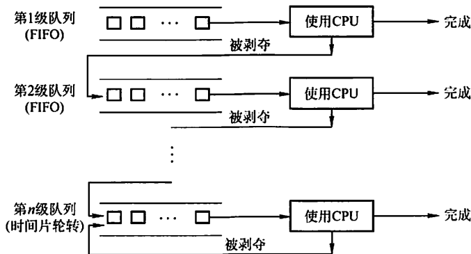
图 2.9 多级反馈队列调度算法
