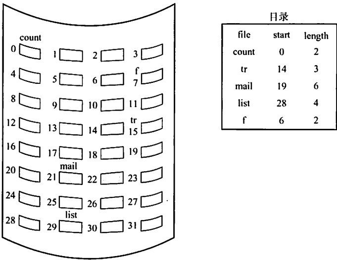
图 4.6 连续分配
