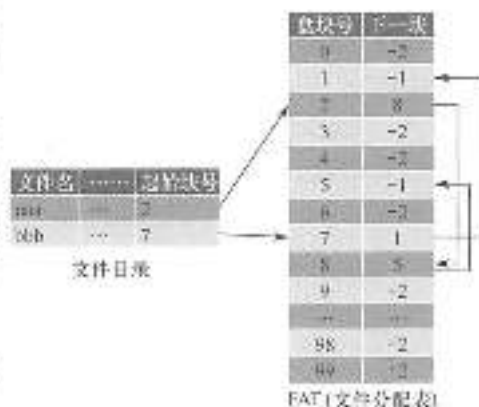
图 4.8 文件分配表
