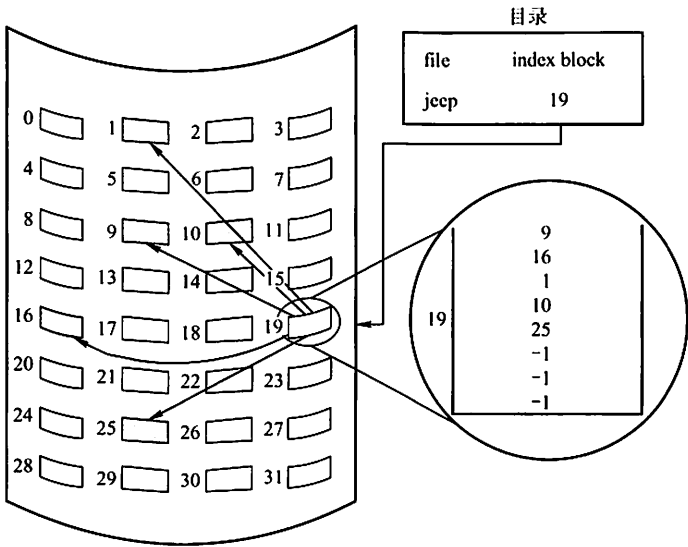
图 4.9 索引分配
