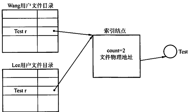
图 4.15 基于索引结点的共享方式
