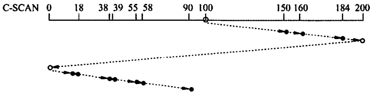
图 5.19 C-SCAN 磁盘调度算法
