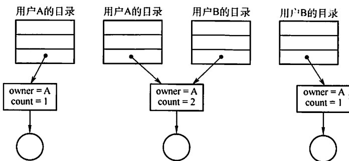
图 4.16 文件共享中的链接计数
