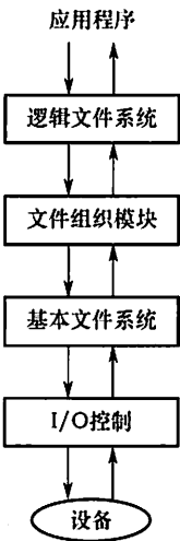
图 4.17 合理的文件系统层次结构
