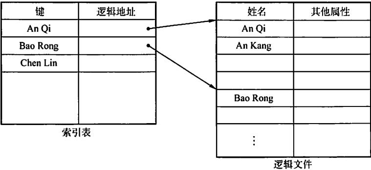
图 4.5 索引顺序文件示意图
