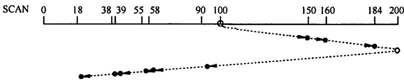
图 5.18 SCAN 磁盘调度算法
