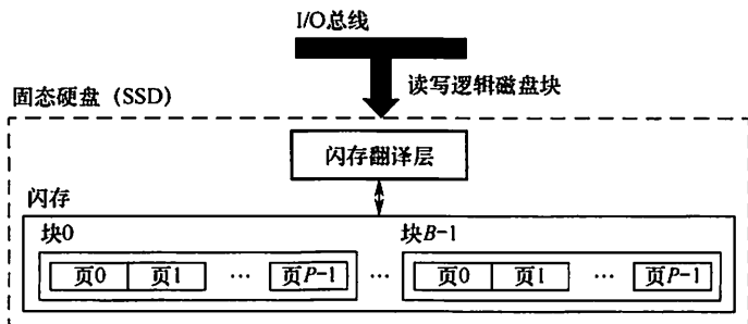
图 5.23 固态硬盘 (SSD)
