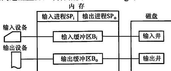
图 5.12 SPOOLing 系统的组成
