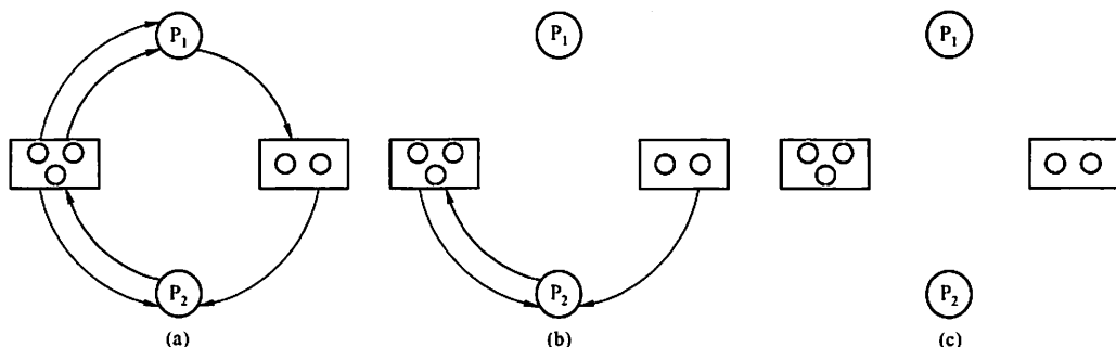
图 2.16 资源分配图的化简
