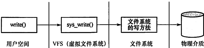
图 4.23 write() 系统调用操作示意图
