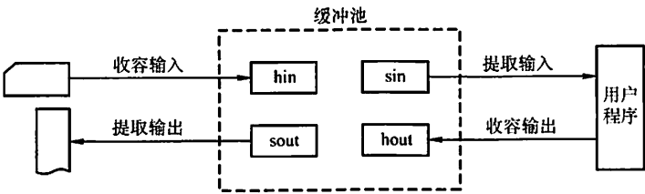
图 5.9 缓冲池的工作方式
