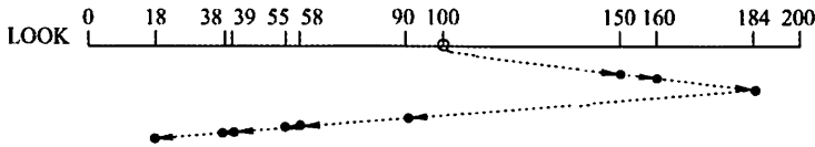
图 5.20 LOOK 磁盘调度算法
