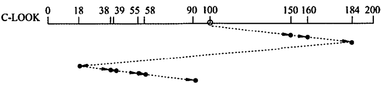
图 5.21 C-LOOK 磁盘调度算法
