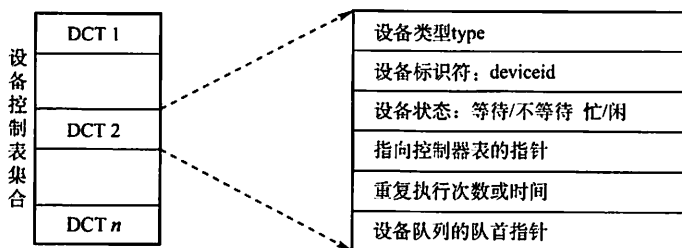
图 5.10 设备控制表 DCT
