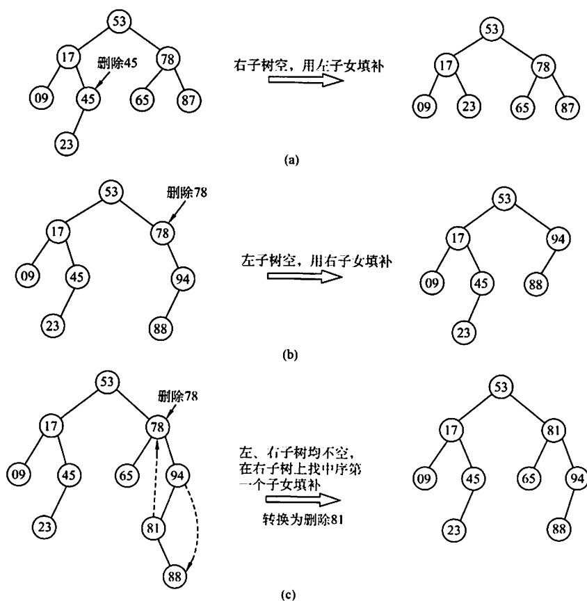
图 7.7 3 种情况下的删除过程
