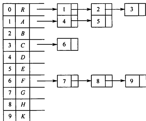
(a) 孩子表示法
