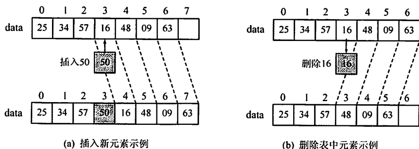
图 2.2 顺序表的插入和删除
