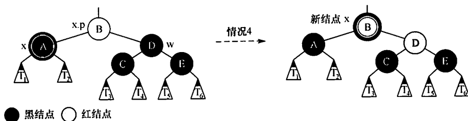
图 7.26 情况 4 的调整方式
