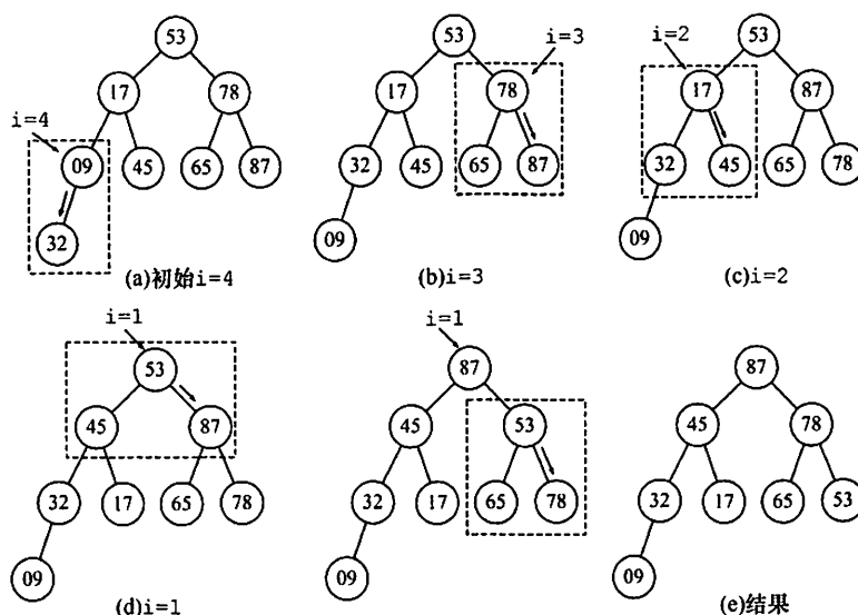
图 8.5 自下往上逐步调整为大根堆
