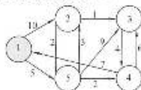
图 6.17 应用 Dijkstra 算法图
