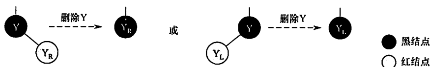
图 7.22 只有右子树或左子树的删除情况
