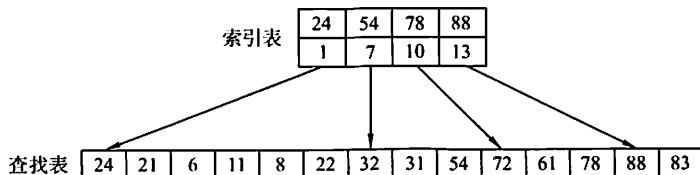
图 7.3 分块查找示意图
