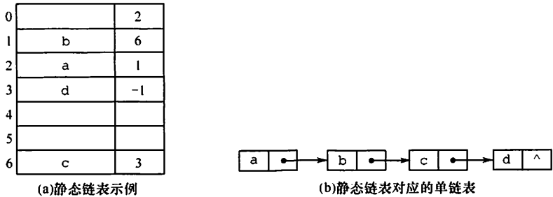
图 2.14 静态链表存储示意图
