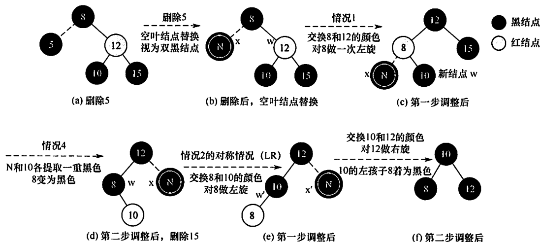
图 7.27 红黑树的删除过程
