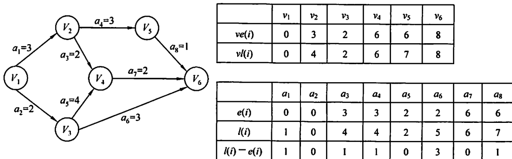
图 6.23 求解关键路径的过程
