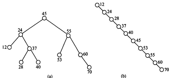
图 7.8 相同关键字组成的不同二叉排序树
