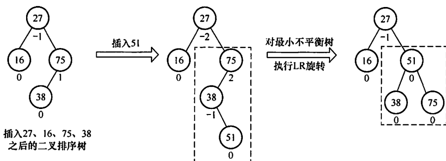
图 7.10 最小不平衡子树示意
