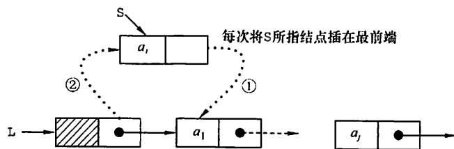
图 2.5 头插法建立单链表
