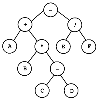
图 3.15 A+B*(C-D)-E/F 对应的表达式树
