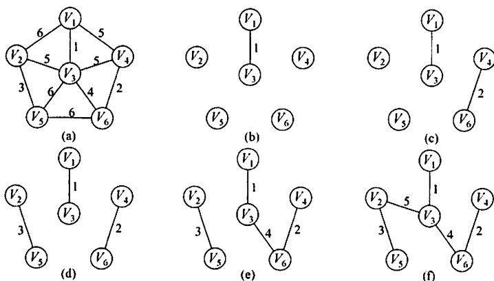
图 6.16 Kruskal 算法构造最小生成树的过程
