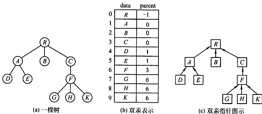
图 5.14 树的双亲表示法
