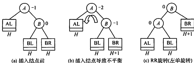
图 7.12 RR 平衡旋转
