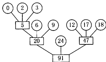
图 8.18 8个归并段的最佳归并树
