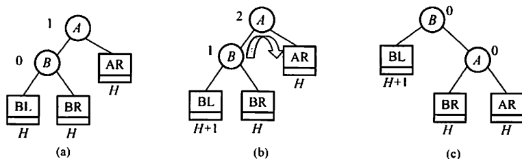
图 7.11 LL 平衡旋转
