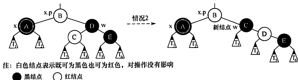
图 7.24 情况 2 的调整方式
