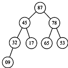
图 8.4 一个大根堆示意图
