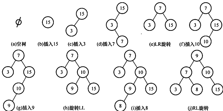
图 7.15 平衡二叉树的生成过程
