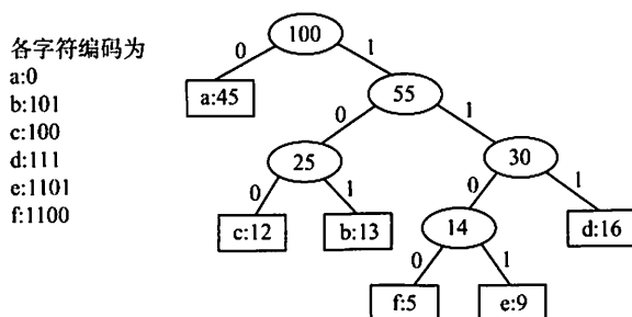
图 5.20 由哈夫曼树构造哈夫曼编码
