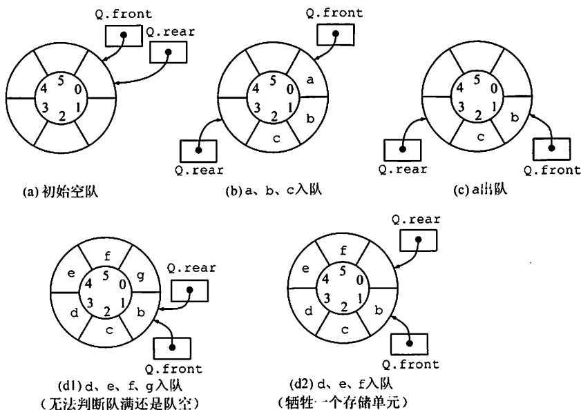
图 3.7 循环队列出入队示意图
