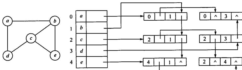
图 6.10 无向图的邻接多重表表示
