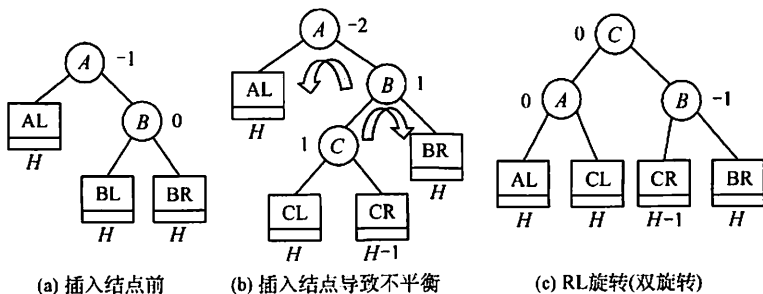
图 7.14 RL 平衡旋转
