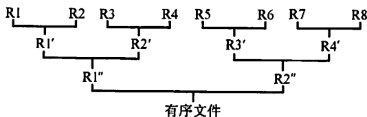
图 8.13 2 路平衡归并的排序过程
