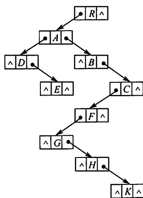
(b) 孩子兄弟表示法
