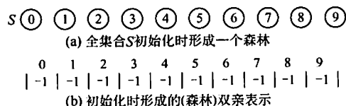
图 5.21 并查集的初始化
