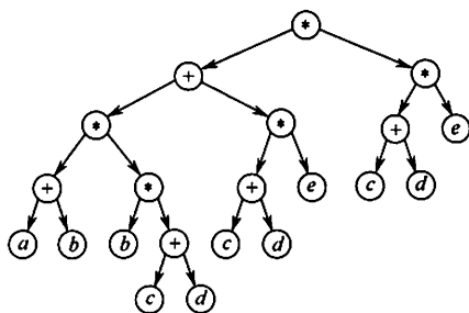
图 6.20 二叉树描述表达式
