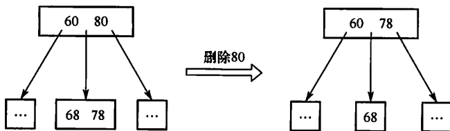
图 7.30 B 树中删除非终端结点关键字的取代
