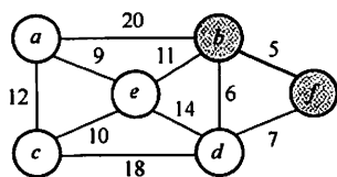
第一步 选取边 \langle b, f \rangle
