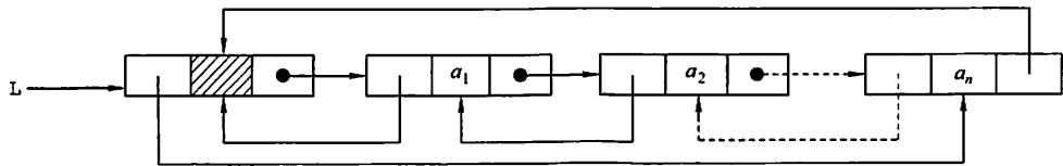
图 2.13 循环双链表
