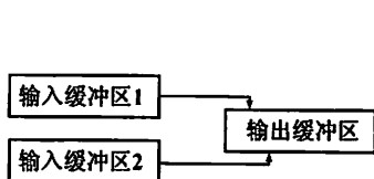
图 8.12 2 路归并
