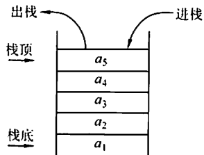
图 3.1 栈的示意图
