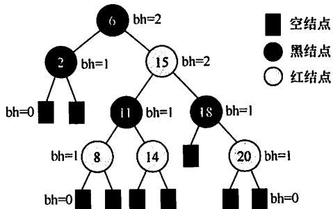
图 7.18 一棵红黑树
