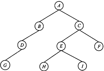
图 3.17 二叉树
