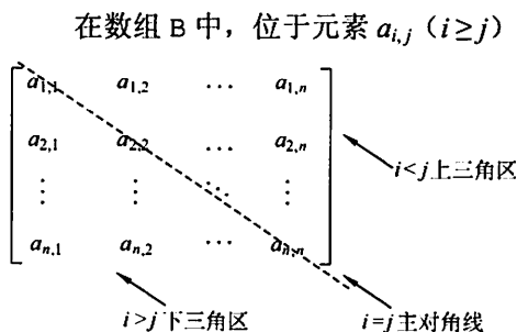
图 3.20 n 阶方阵的划分
