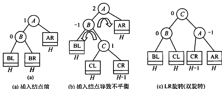
图 7.13 LR 平衡旋转
