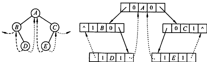
图 5.11 中序线索二叉树及其二叉链表表示
