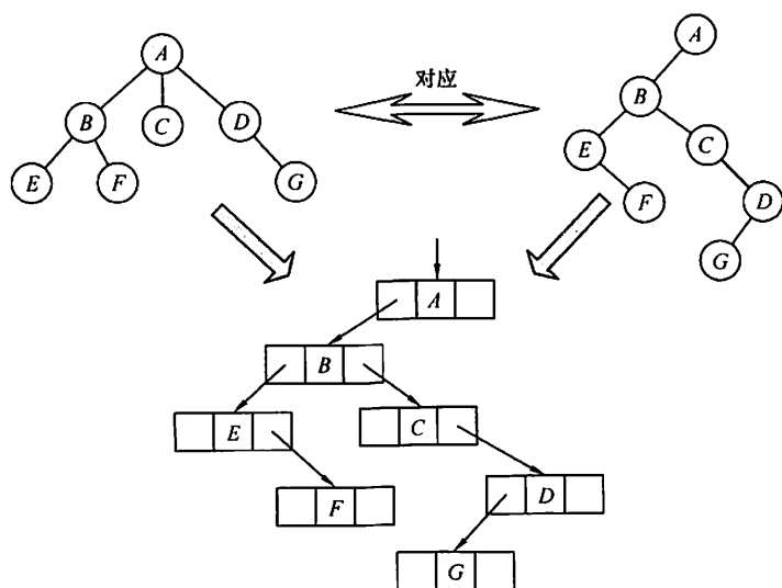
图 5.16 树与二叉树的对应关系
