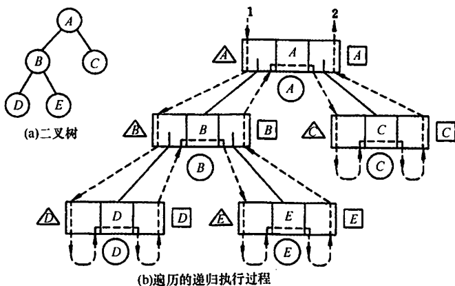
图 5.7 三种遍历过程示意图
