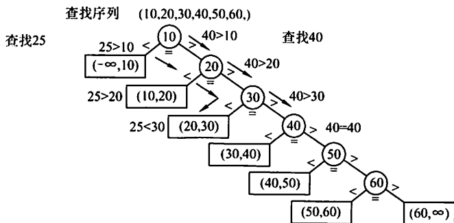
图 7.1 有序顺序表上的顺序查找判定树
