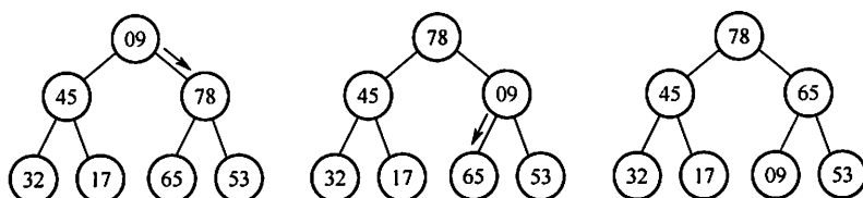
图 8.6 输出堆顶元素后再将剩余元素调整成新堆
