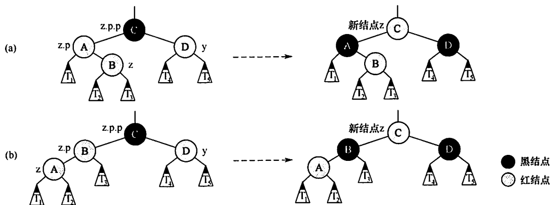
图 7.20 情况3的调整方式
