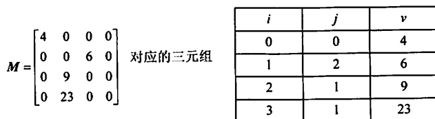
图 3.26 稀疏矩阵及其对应的三元组
