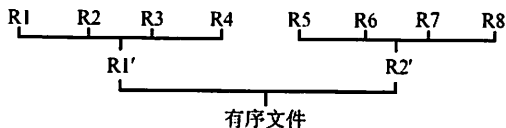
图 8.14 4 路平衡归并的排序过程
