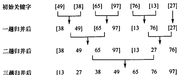
图 8.8 2路归并排序示例
