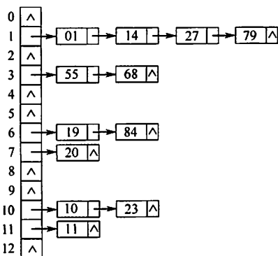
图 7.33 拉链法处理冲突的散列表
