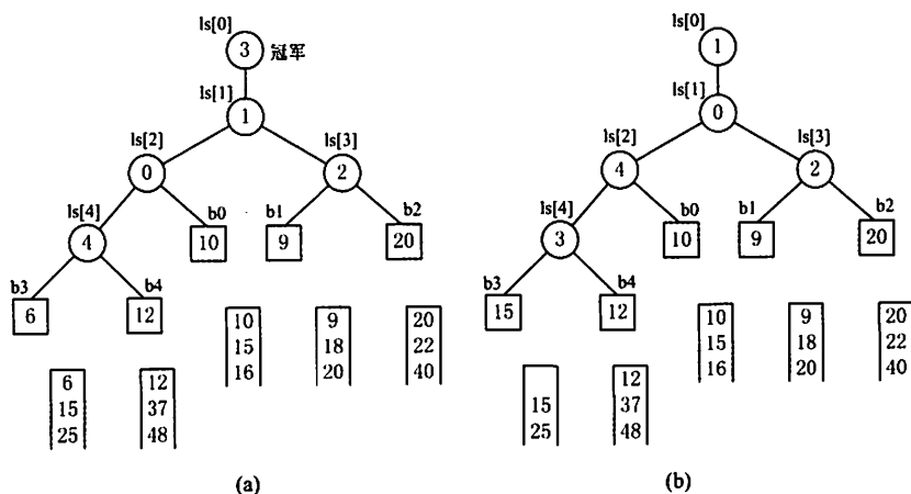
图 8.15 实现 5 路归并的败者树
