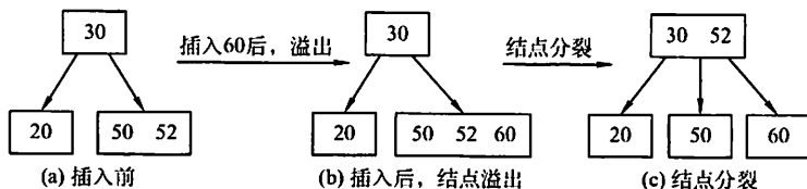
图 7.29 结点的“分裂”示意
