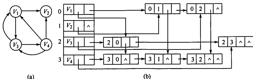
图 6.9 有向图的十字链表表示
