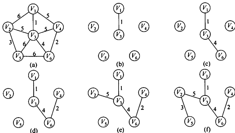
图 6.15 Prim 算法构造最小生成树的过程
