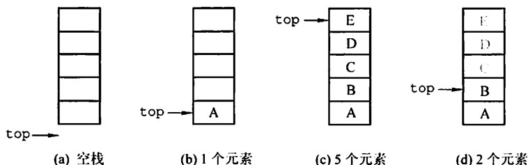
图 3.2 栈顶指针和栈中元素之间的关系
