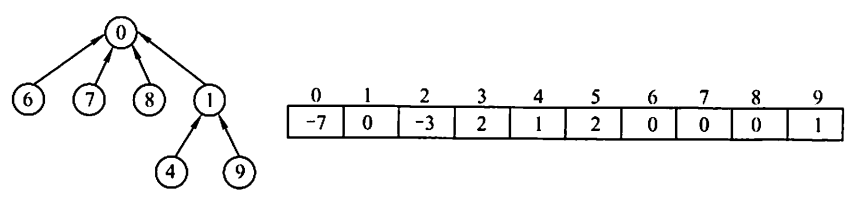
图 5.22 用树表示并查集
