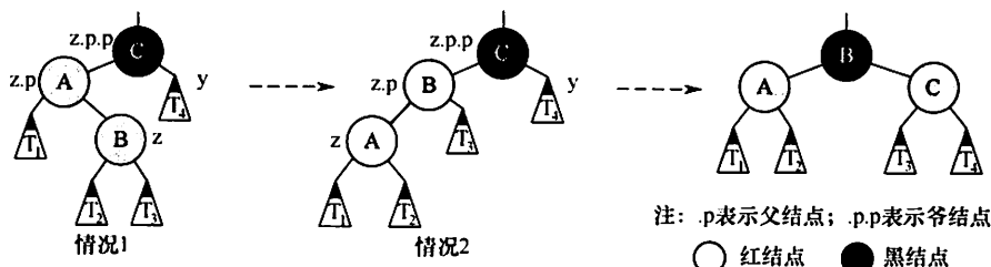
图 7.19 情况 1 和情况 2 的调整方式
