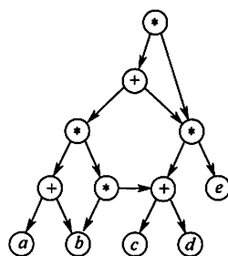
图 6.21 有向无环图描述表达式
