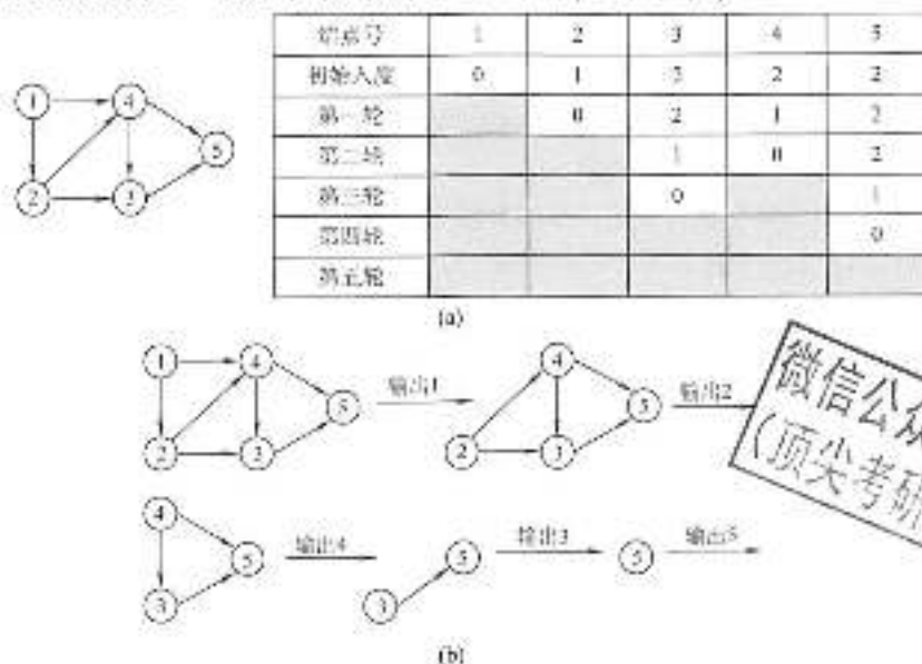
图 6.22 有向无环图的拓扑排序过程
