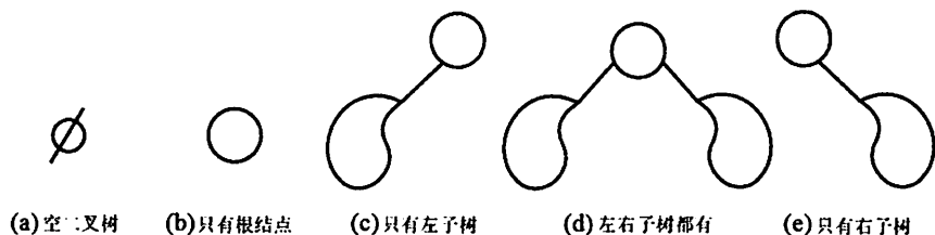
图 5.2 二叉树的 5 种基本形态
