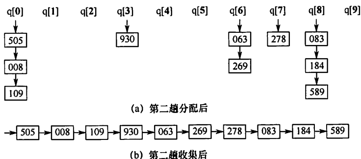
图 8.10 第二趟链式基数排序操作
