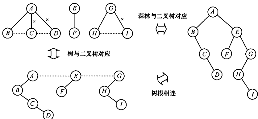
图 5.17 森林与二叉树的对应关系
