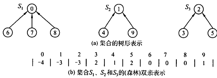
图 5.22 用树表示并查集
