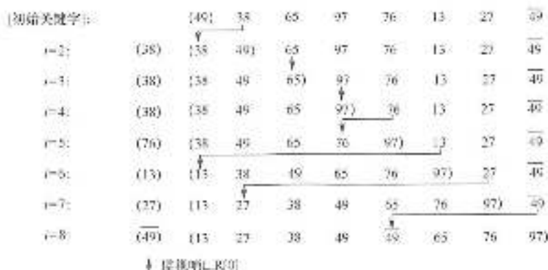
图 8.1 直接插入排序示例
