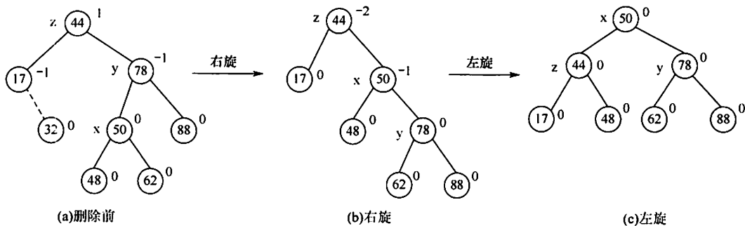
图 7.16 平衡二叉树的删除
