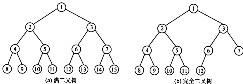
图 5.3 两种特殊形态的二叉树 ①
