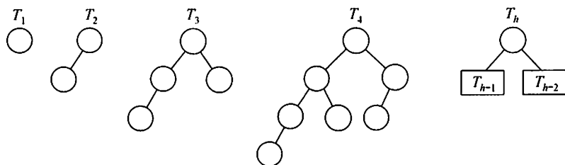
图 7.17 结点数 n 最少的平衡二叉树
