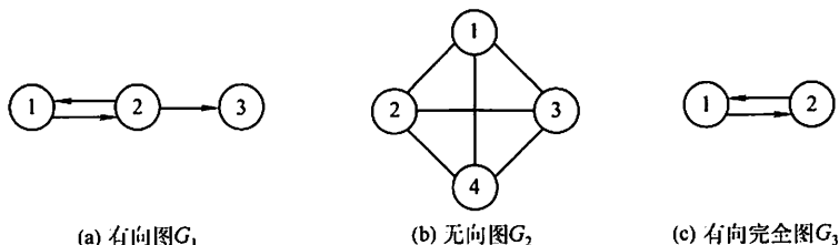
图 6.1 图的示例
