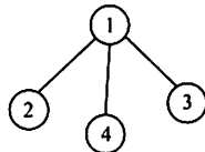
图 6.4 图 G_2 的一个生成树
