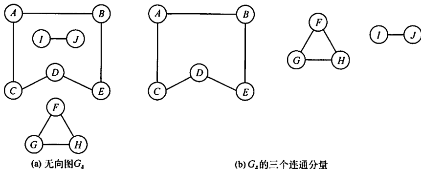
图 6.2 无向图及其连通分量
