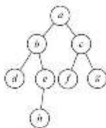
图 6.11 一个无向图 G
