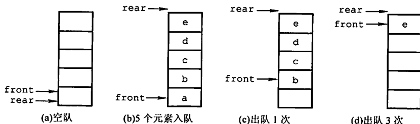
图 3.6 队列的操作
