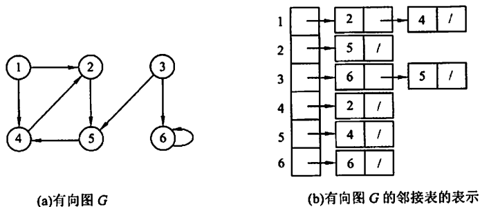
图 6.8 有向图邻接表表示法实例
