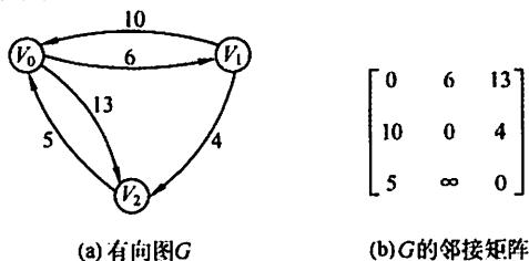
图 6.19 带权有向图 G 及其邻接矩阵
