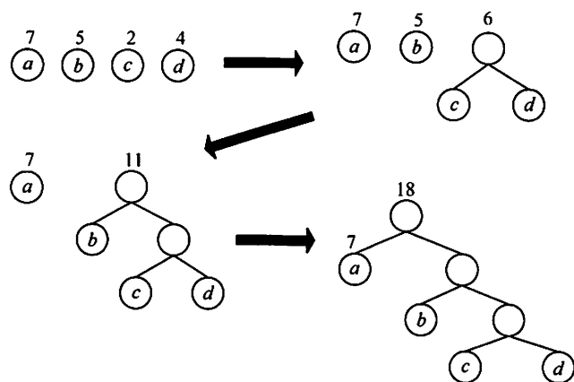
图 5.19 哈夫曼树的构造过程
