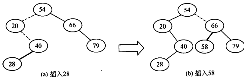
图 7.5 向二叉排序树中插入结点
