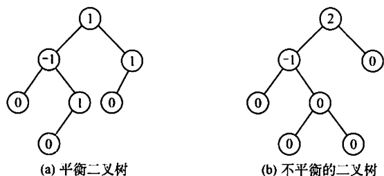
图 7.9 平衡二叉树和不平衡的二叉树
