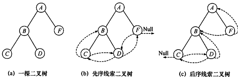
图 5.13 先序线索二叉树和后序线索二叉树
