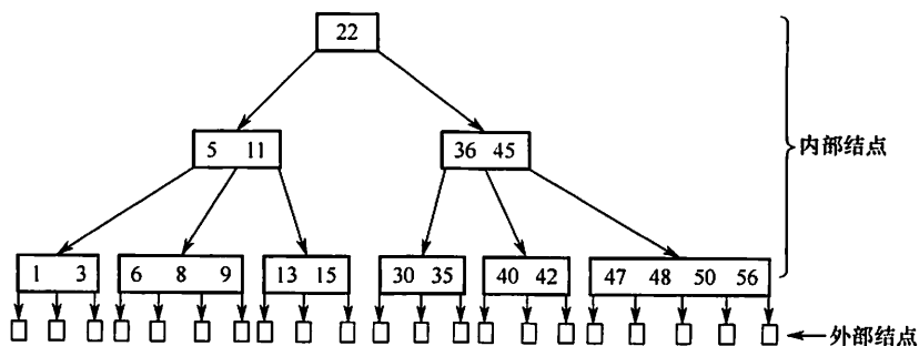
图 7.28 一棵 5 阶 B 树的实例
