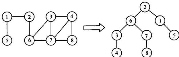
图 6.12 图的广度优先生成树
