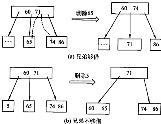
图 7.31 B 树中删除终端结点关键字的示意图
