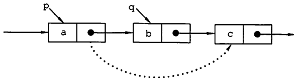
图 2.8 单链表结点的删除
