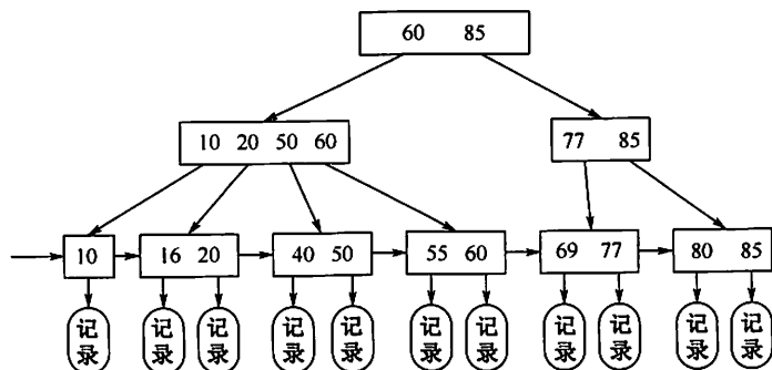
图 7.32 B+树结构示意图
