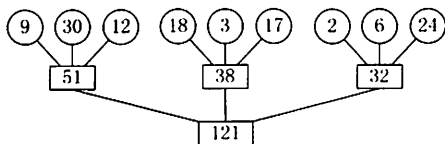
图 8.16 3路平衡归并的归并树
