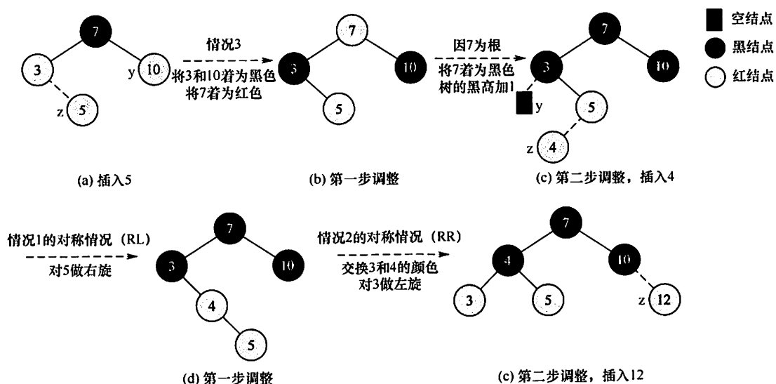
图 7.21 红黑树的插入过程
