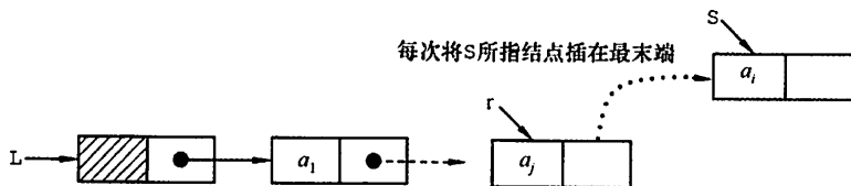
图 2.6 尾插法建立单链表
