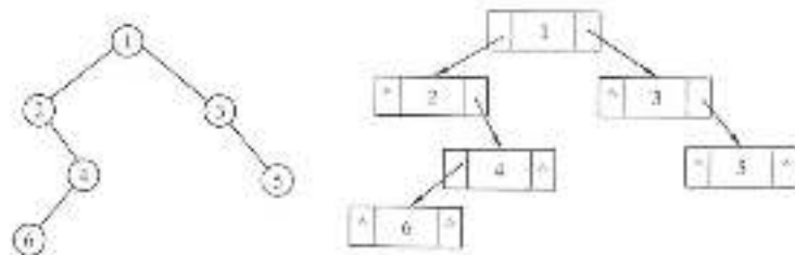
图 5.6 二叉链表的存储结构
