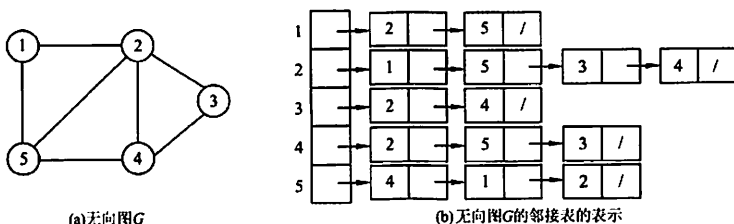
图 6.7 无向图邻接表表示法实例
