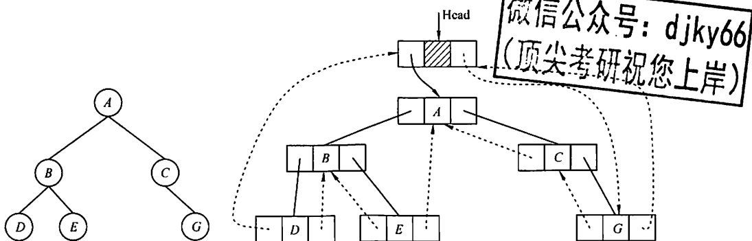
图 5.12 带头结点的中序线索二叉树
