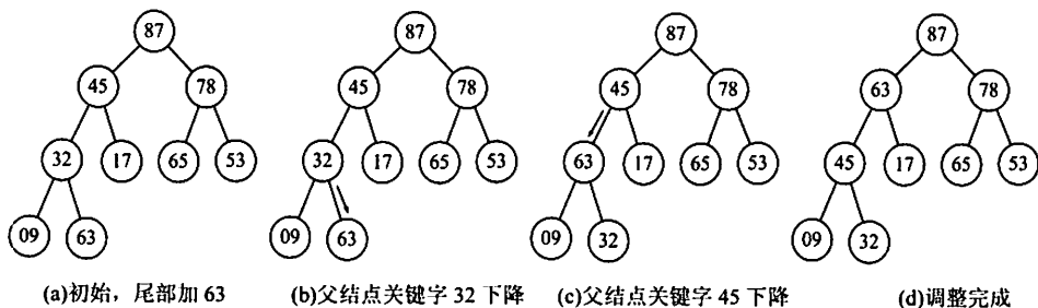
图 8.7 大根堆的插入操作示例
