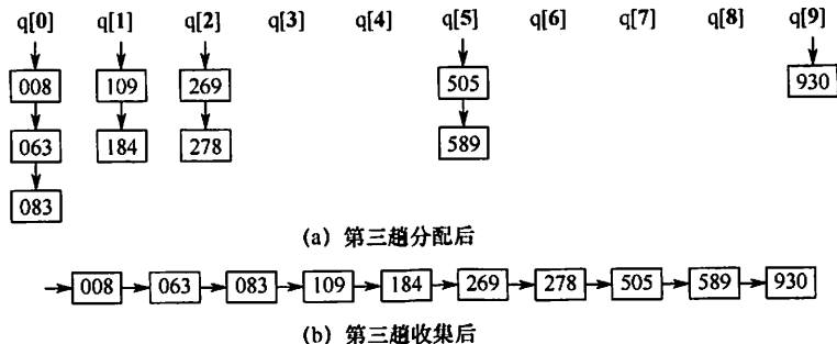
图 8.11 第三趟链式基数排序操作
