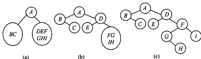
图 5.9 一棵二叉树的构造过程
