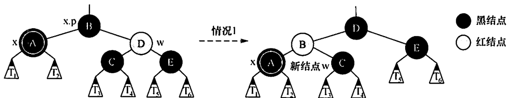
图 7.23 情况 1 的调整方式
