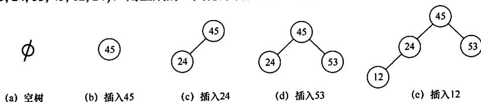
图 7.6 二叉排序树的构造过程
