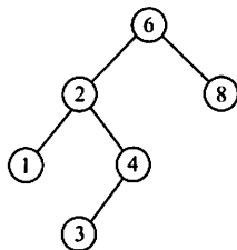
图 7.4 一棵二叉排序树
