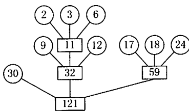
图 8.17 3路平衡归并的最佳归并树
