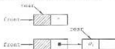
图 3.9 带头结点的链式队列
