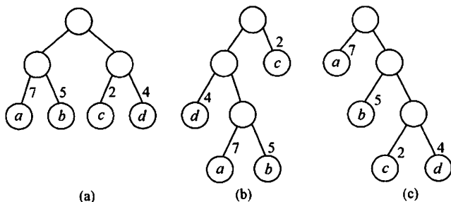
图 5.18 具有不同带权长度的二叉树
