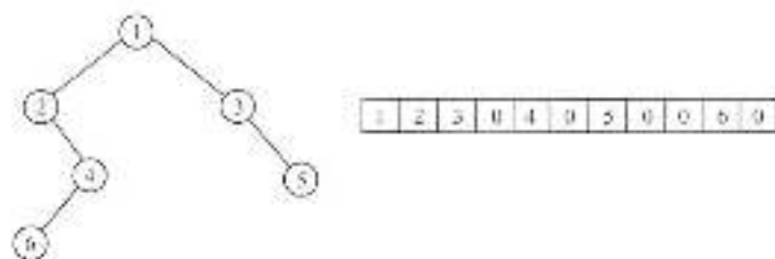
图 5.4 二叉树的顺序存储结构
