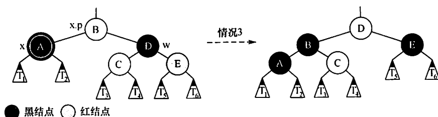
图 7.25 情况 3 的调整方式
