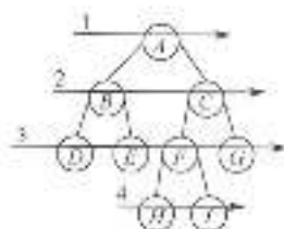
图 5.8 二叉树的层次遍历
