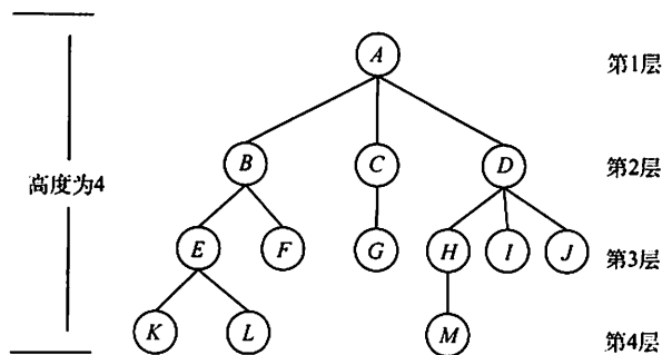
图 5.1 树的树形表示
