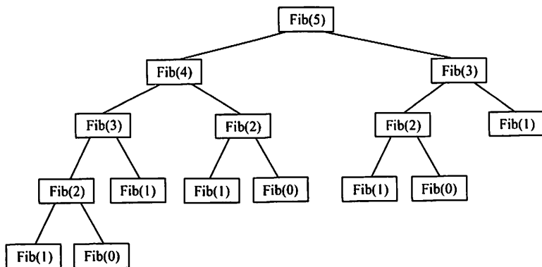
图 3.16 Fib(5)的递归执行过程
