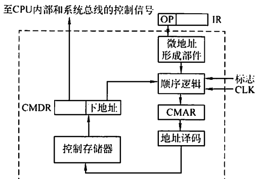
图 5.11 微程序控制器的基本结构
