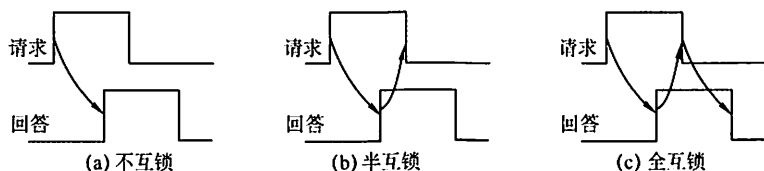
图 6.4 请求和回答信号的互锁
