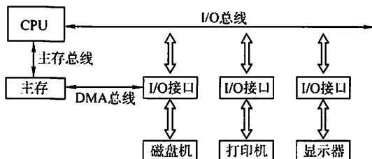
图 6.3 三总线结构
