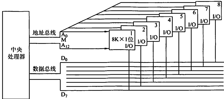
图 3.12 位扩展连接示意图
