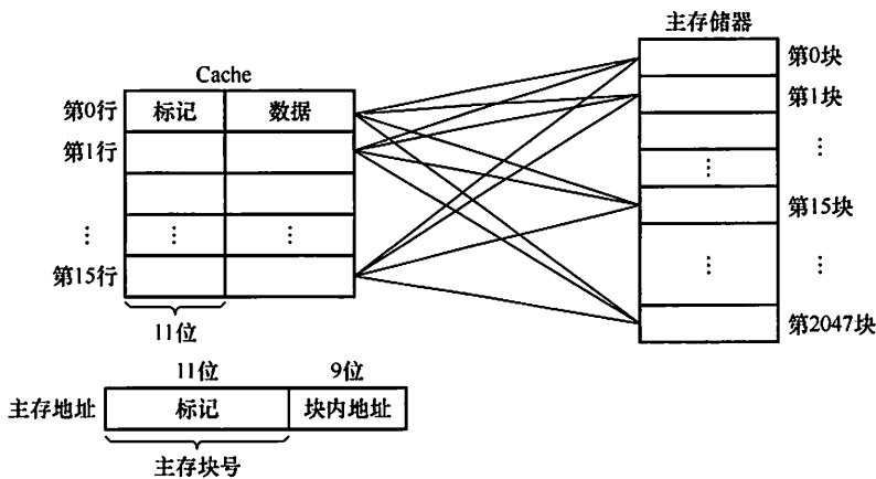
图 3.19 Cache 和主存之间的全相联映射方式
