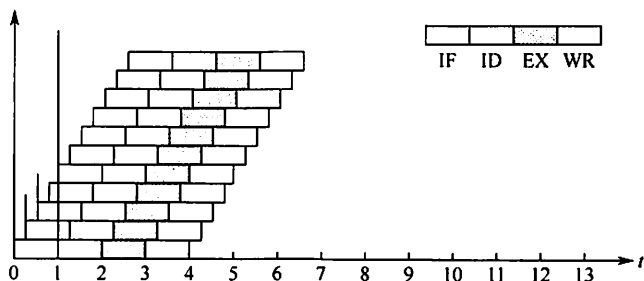
图 5.21 超流水线技术
