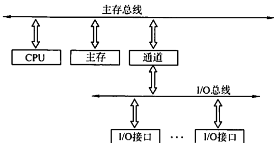
图 6.2 双总线结构
