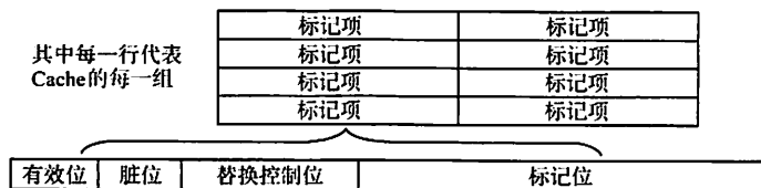
图 3.21 二路组相联的标记阵列示意图
