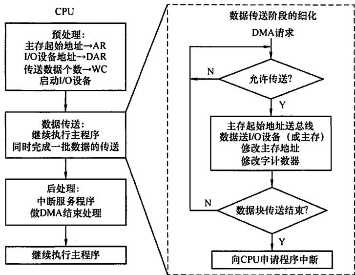
图 7.9 DMA 的传送流程
