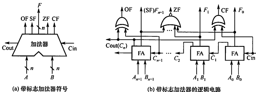
图 2.6 用全加器实现 n 位带标志加法器的电路
