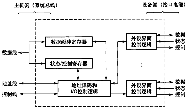
图 7.1 I/O 接口的基本结构
