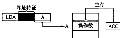
图 4.4 直接寻址
