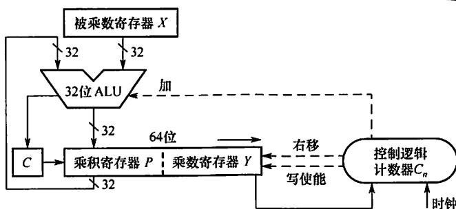
图 2.11 32 位无符号数乘法运算的逻辑结构图
