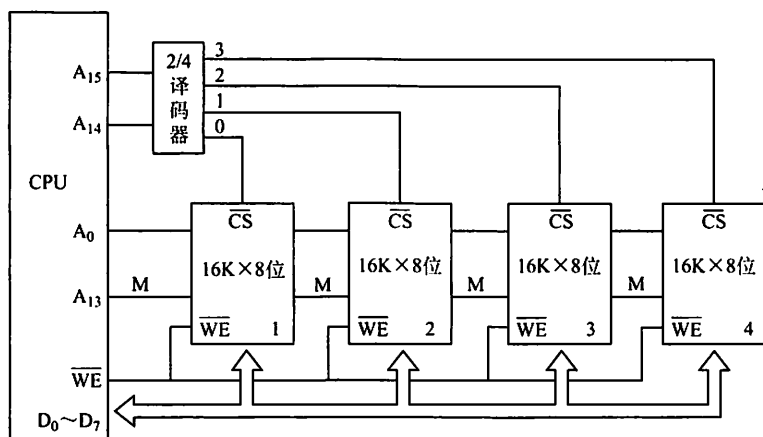
图 3.13 字扩展连接示意图
