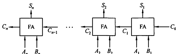
图 2.4 n 位串行进位加法器
