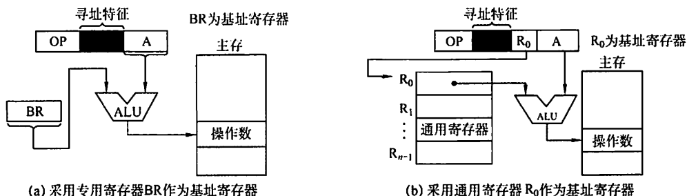
图 4.9 基址寻址
