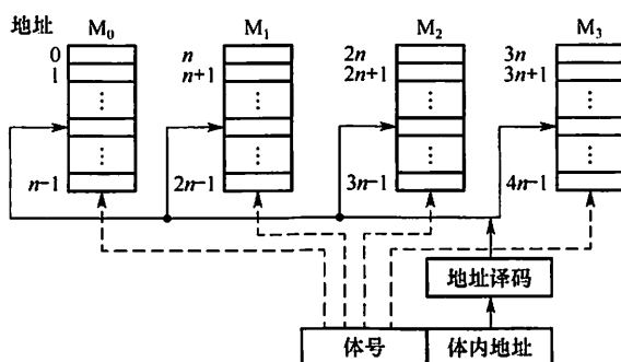
图 3.7 高位交叉编址的多体存储器
