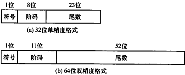
图 2.19 IEEE 754 标准浮点数的格式
