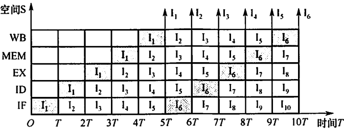
图 5.17 一个 5 段指令流水线时空图
