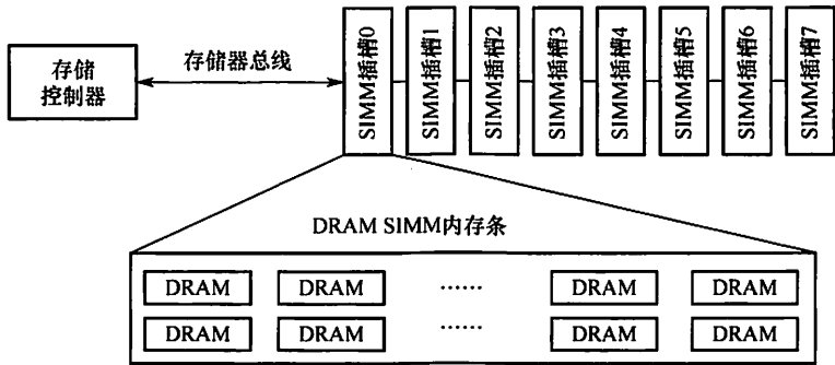
图 3.11 存储控制器、存储器总线和内存条之间的连接关系示意图
