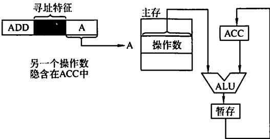
图 4.2 隐含寻址
