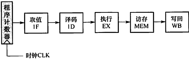
图 5.18 单周期处理机的逻辑构架图
