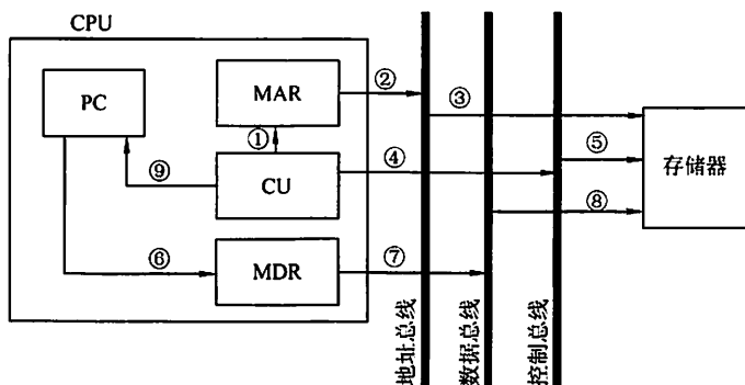
图 5.6 中断周期的数据流
