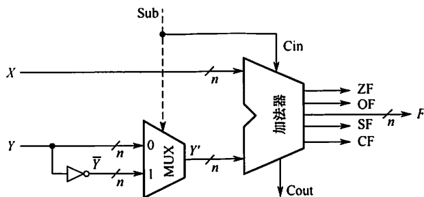
图 2.10 补码加减运算部件
