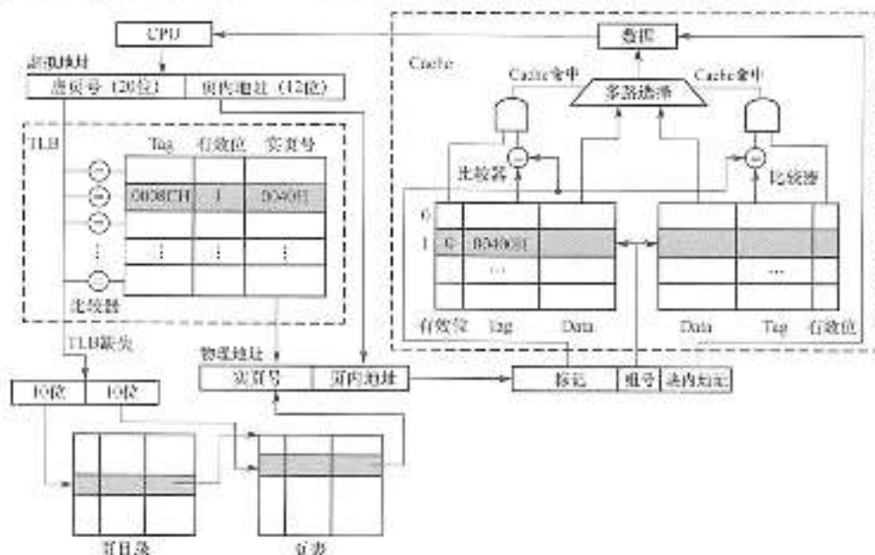
图 3.27 TLB 和 Cache 的访问过程
