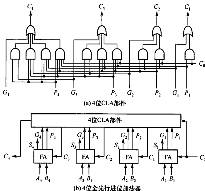
图 2.5 4 位 CLA 部件和 4 位全先行进位加法器
