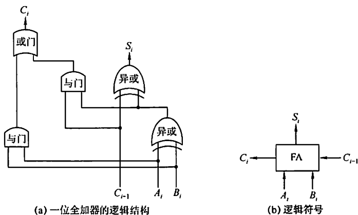
图 2.3 一位全加器
