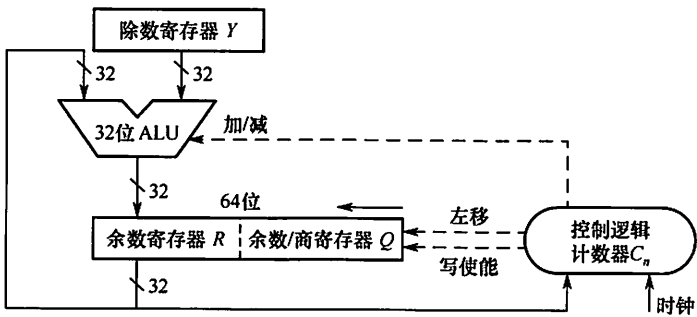
图 2.13 32 位除法运算的逻辑结构图
