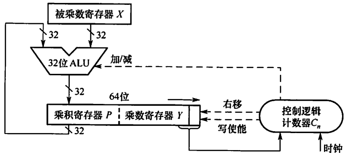
图 2.12 补码一位乘法的逻辑结构图
