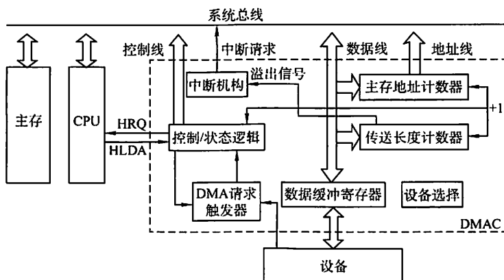
图 7.8 简单的 DMA 控制器
