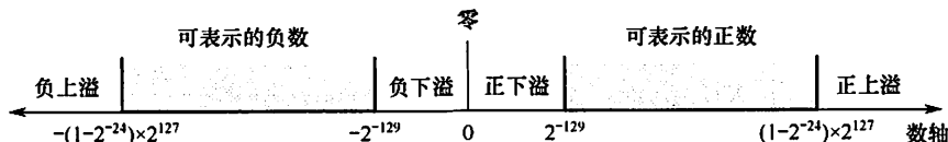
图 2.18 浮点数的表示范围
