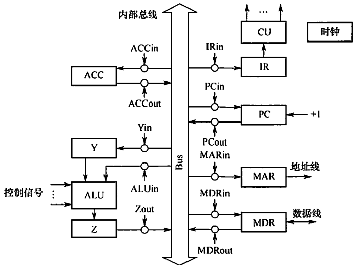
图 5.7 CPU 内部总线的数据通路和控制信号
