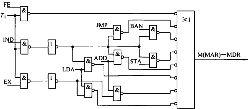
图 5.10 产生 M(MAR) \rightarrow MDR 命令的逻辑图
