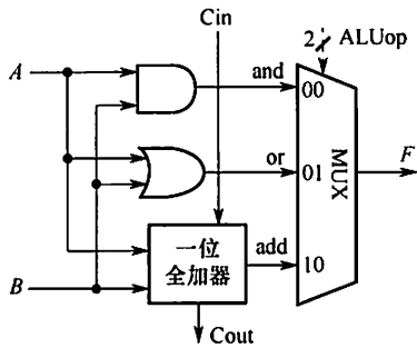
图 2.8 一位 ALU 的结构
