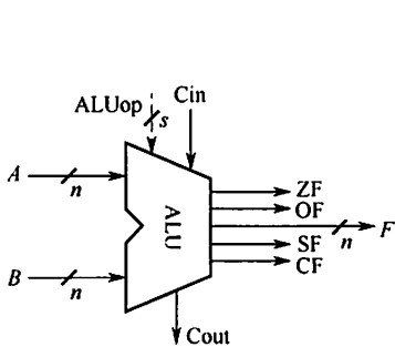
图 2.7 ALU 的基本结构
