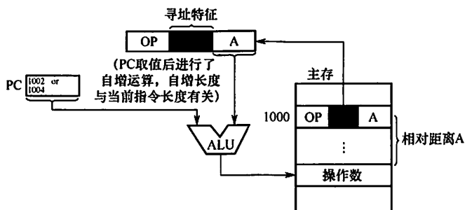
图 4.8 相对寻址
