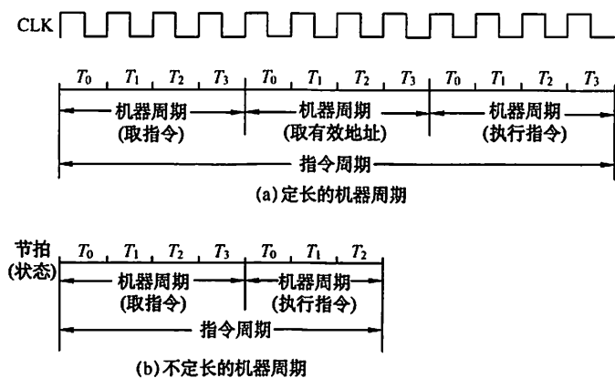
图 5.2 指令周期、机器周期、节拍和时钟周期的关系
