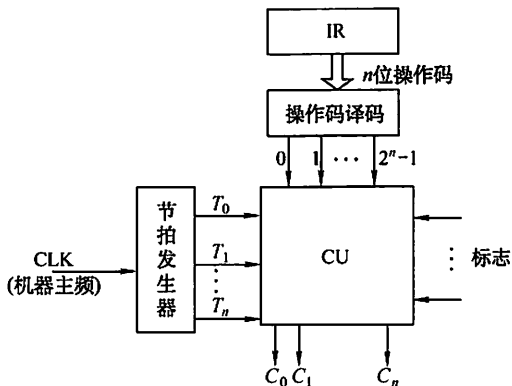
图 5.9 带指令译码器和节拍输入的控制单元图
