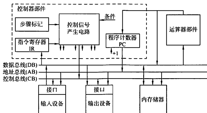
图 5.8 计算机硬件系统和控制器部件的组成
