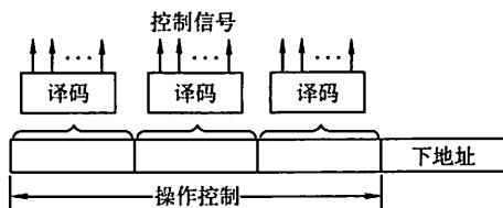
图 5.13 微指令的字段直接编码方式
