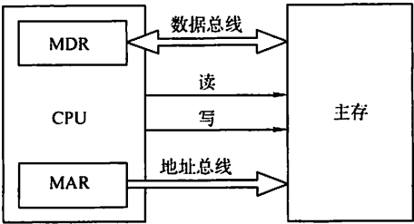
图 3.10 主存储器与 CPU 的连接
