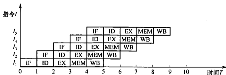
图 5.16 一个 5 段指令流水线
