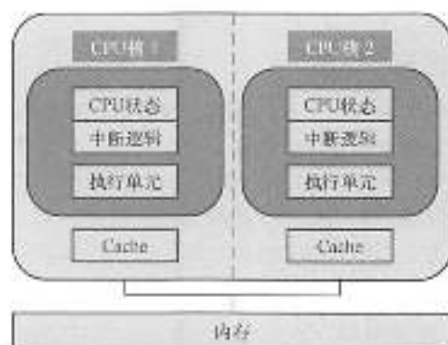
图 5.23 不共享 Cache 的双核 CPU 结构
