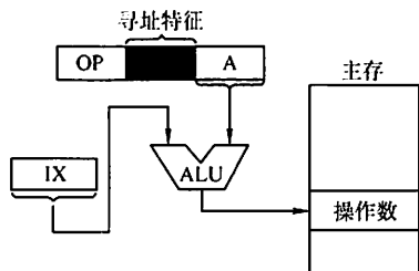
图 4.10 变址寻址
