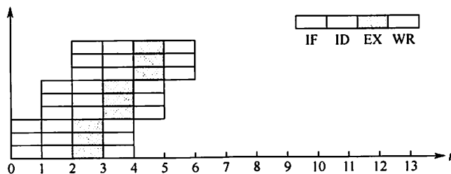
图 5.20 超标量流水线技术
