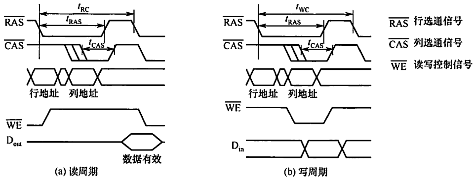
图 3.4 DRAM 芯片读周期时序图
