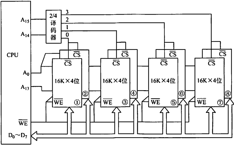
图 3.14 字位同时扩展及 CPU 的连接图
