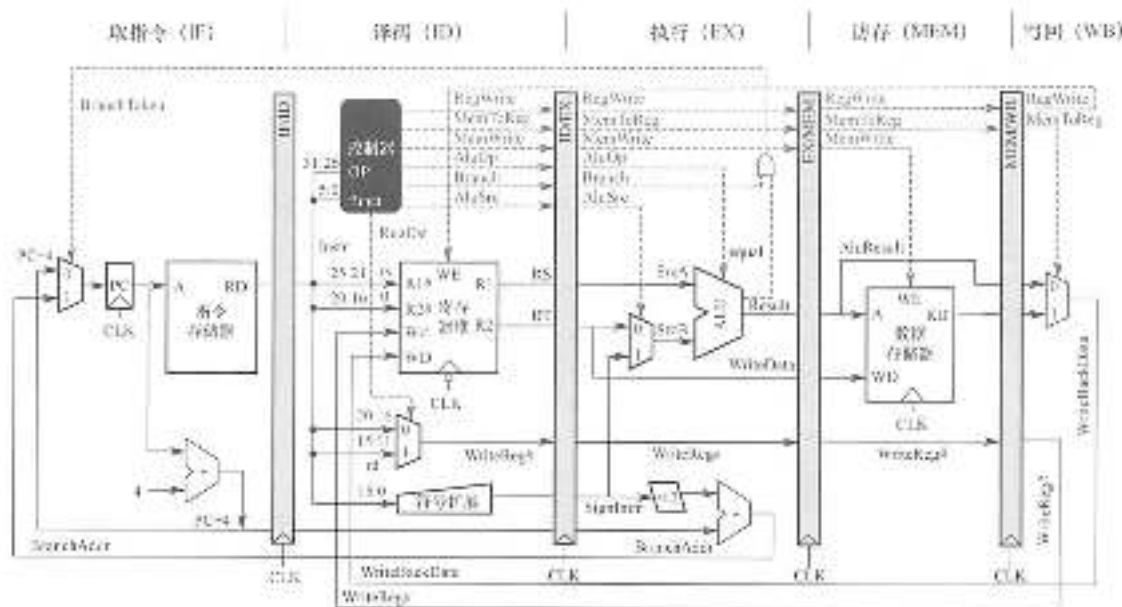
图 5.19 一个 5 段流水线数据通路 (及控制信号)
