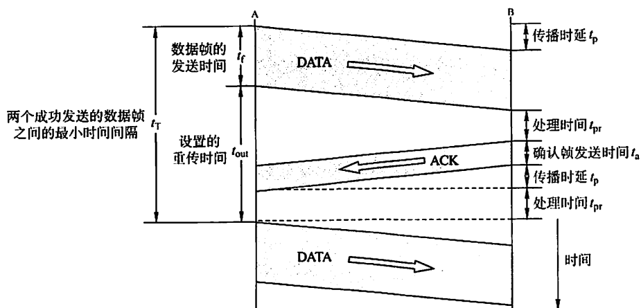
图 3.9 停止-等待协议中数据帧和确认帧的发送时间关系
