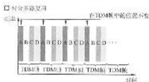
图 3.15 时分多路复用原理示意图
