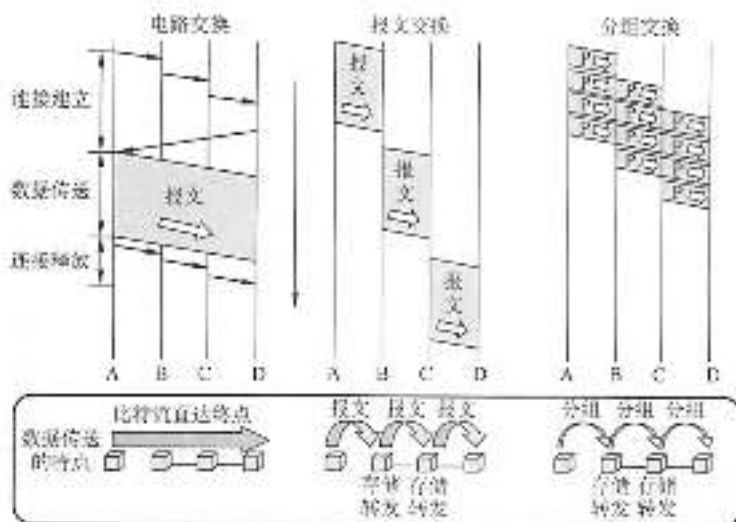
图 2.4 三种数据交换方式的比较
