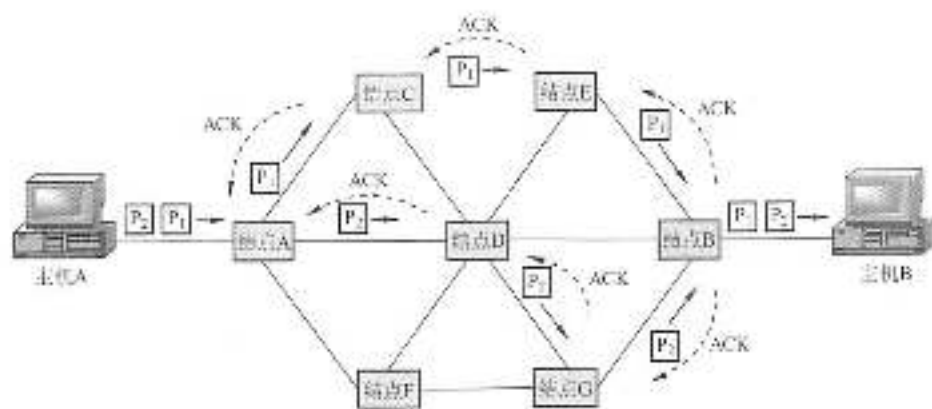
图 2.5 数据报方式转发分组
