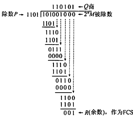
图 3.6 循环冗余码的运算过程
