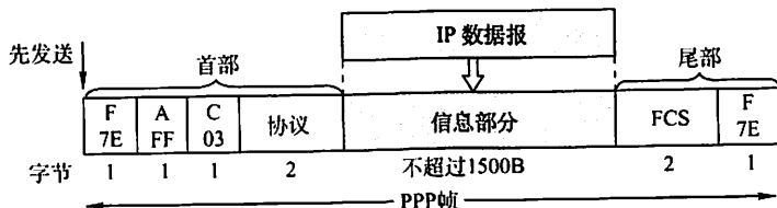
图 3.34 PPP 帧的格式
