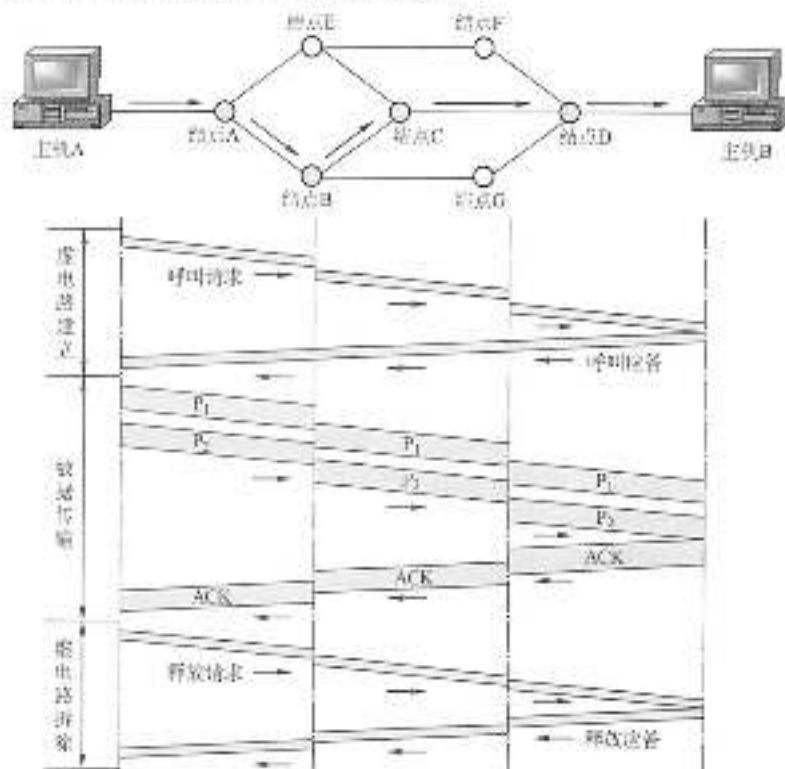
图 2.6 虚电路方式的工作原理
