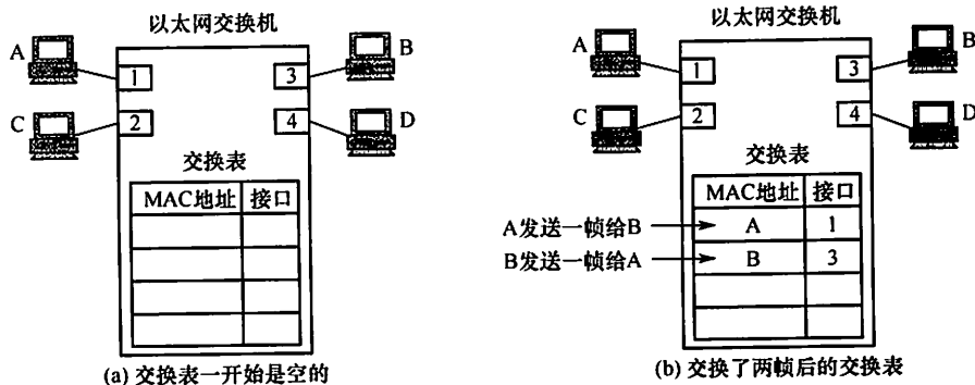
图 3.37 以太网交换机中的交换表
