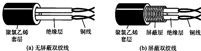
图 2.7 双绞线的结构
