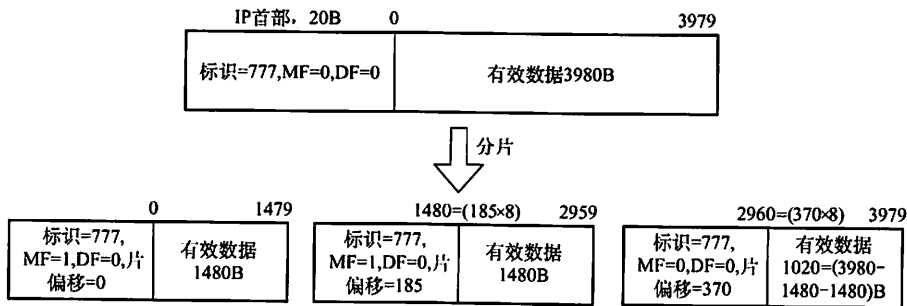
图 4.5 IP 分片的例子
