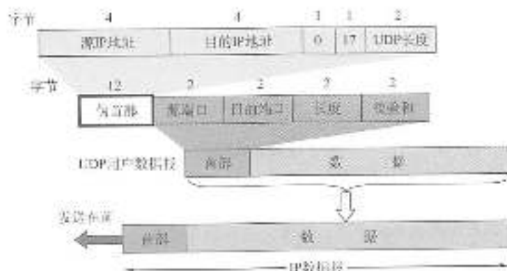
图 5.4 UDP 数据报的首部和伪首部
