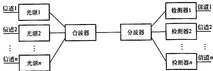
图 3.16 波分多路复用原理示意图
