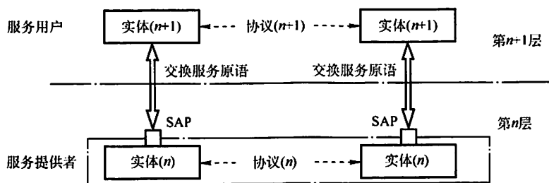
图 1.7 协议、接口、服务三者之间的关系
