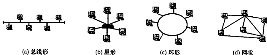
图 1.2 几种不同的网络拓扑结构
