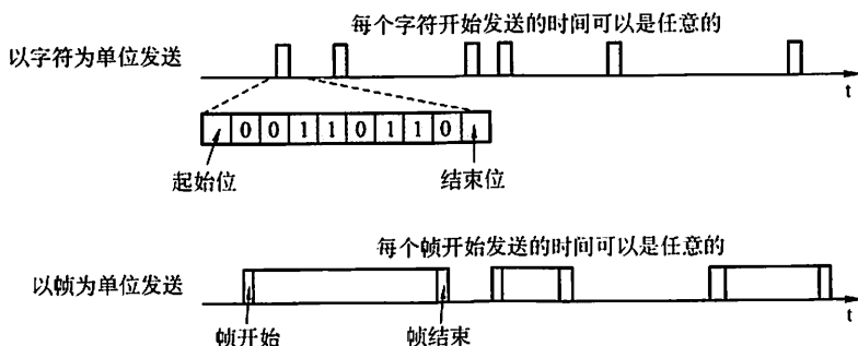
图 2.13 以字符、帧为单位的异步通信
