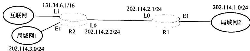
图 4.16 一个简单的网络拓扑
