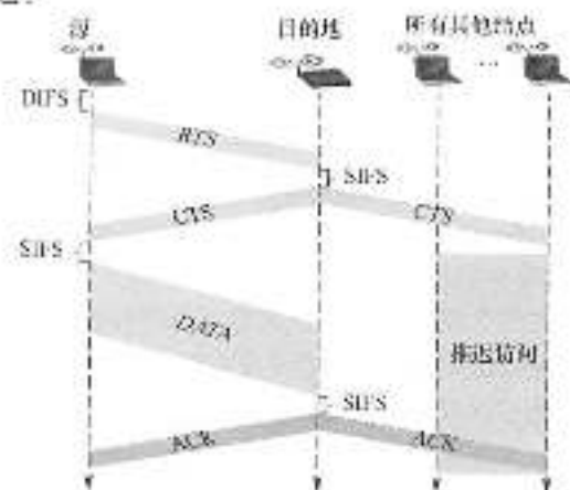
图 3.24 使用 RTS 和 CTS 帧的碰撞避免
