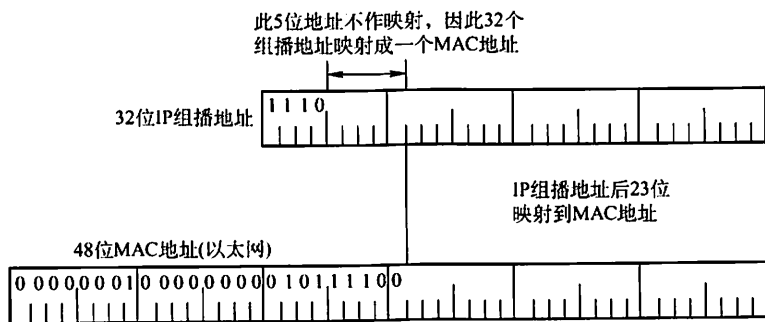
图 4.14 D 类 IP 地址与以太网组播地址的映射关系
