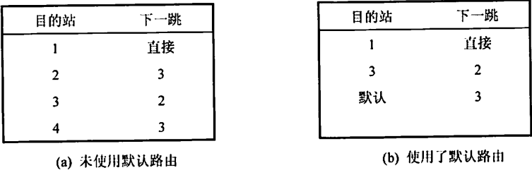
图 4.17 未使用默认路由的转发表和使用了默认路由的转发表的对比
