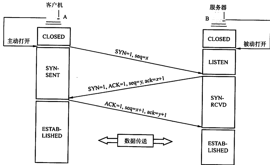
图 5.7 用“三次握手”建立 TCP 连接
