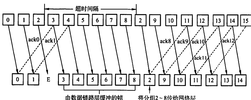
图 3.11 选择重传协议
