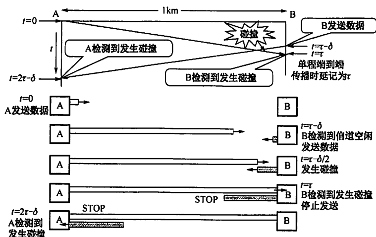
图 3.22 传播时延对载波侦听的影响
