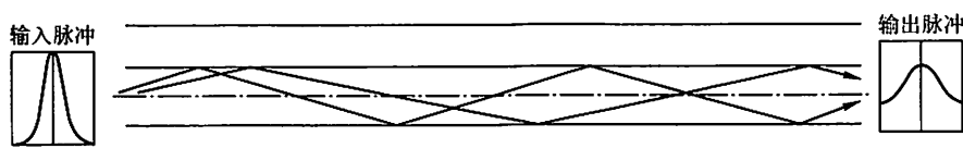
图 2.10 多模光纤
