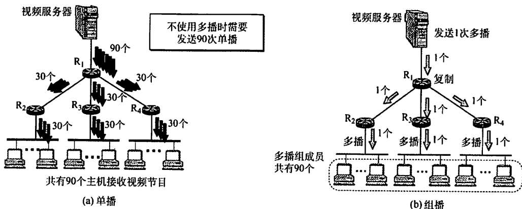
图 4.13 单播与组播的比较
