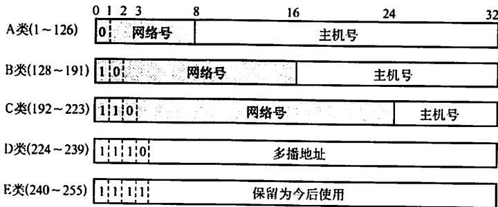
图 4.6 分类的 IP 地址
