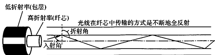
图 2.9 光波在纤芯中的传播
