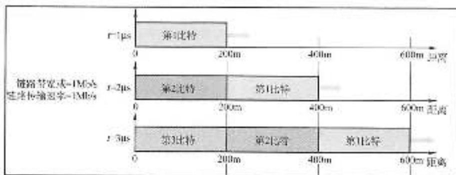
图 1.15 传输速率、带宽和传播速率三者的区别
