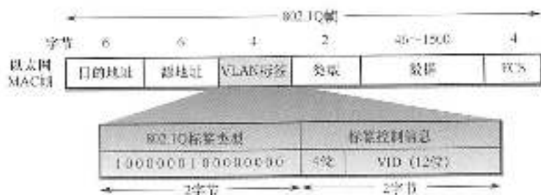
图 3.31 插入 VLAN 标签后变成了 802.1Q 帧
