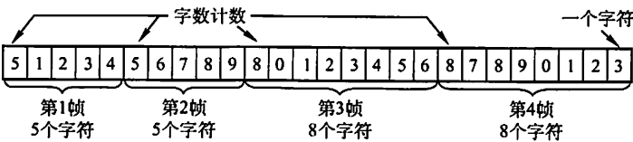
图 3.3 字符计数法
