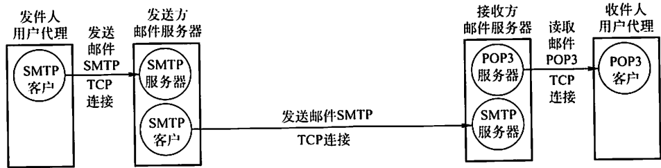
图 6.8 电子邮件系统最主要的组成构件
