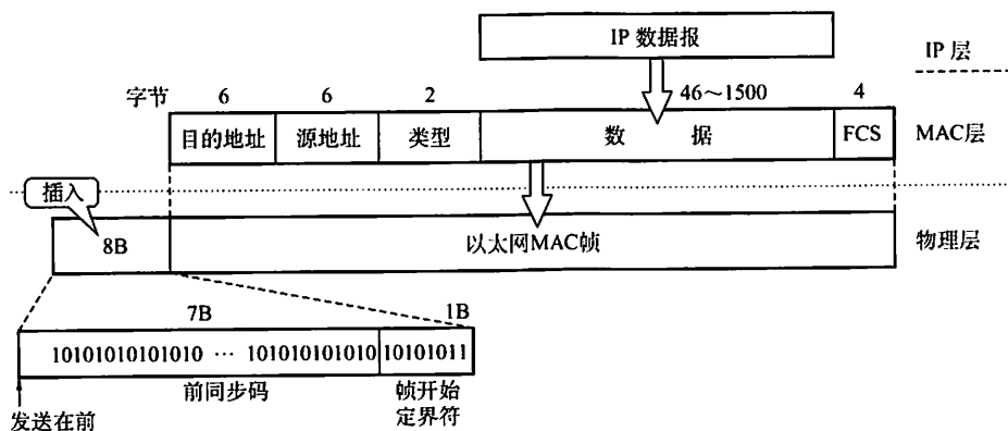
图 3.26 以太网 V2 标准的 MAC 帧格式
