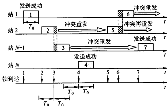
图 3.20 纯 ALOHA 协议的工作原理
