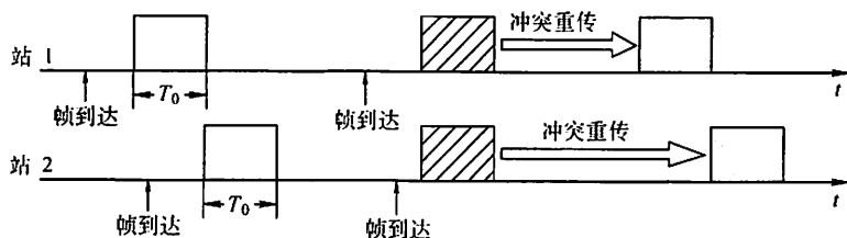
图 3.21 时隙 ALOHA 协议的工作原理
