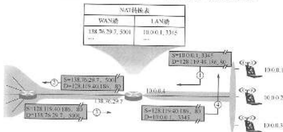
图 4.7 NAT 路由器的工作原理
