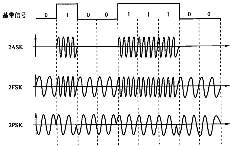
图 2.3 数字调制的三种方式
