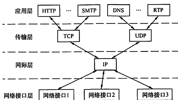
图 1.11 TCP/IP 模型的层次结构及各层的主要协议
