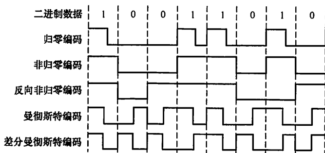
图 2.2 常用的数字数据编码
