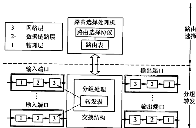
图 4.15 路由器体系结构
