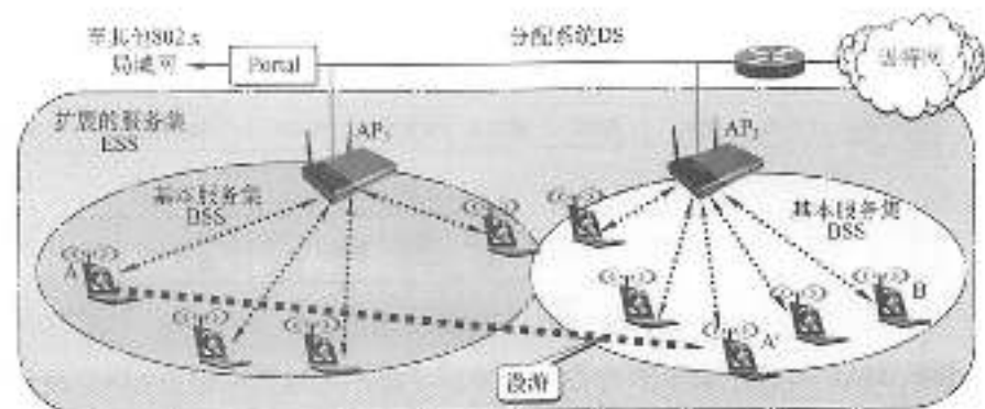
图 3.27 基本服务集和扩展服务集
