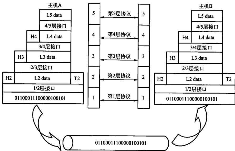
图 1.5 网络各层数据单元的联系
