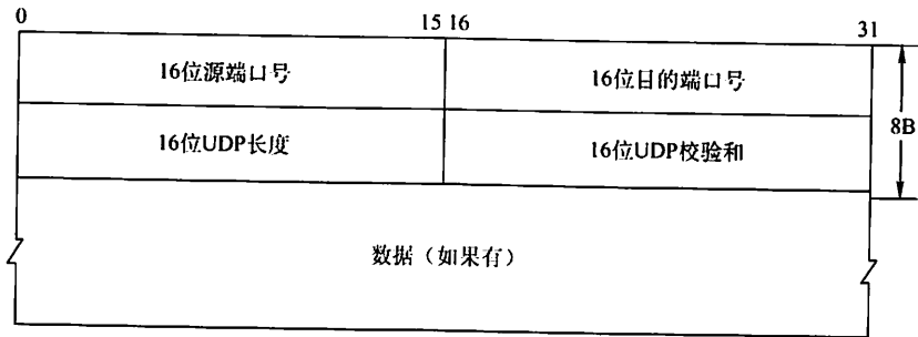
图 5.2 UDP 数据报格式
