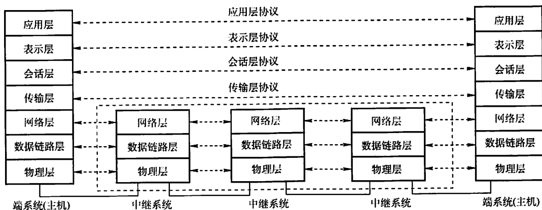
图 1.8 OSI 参考模型的层次结构
