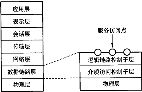
图 3.25 IEEE 802 协议层与 OSI 模型的比较
