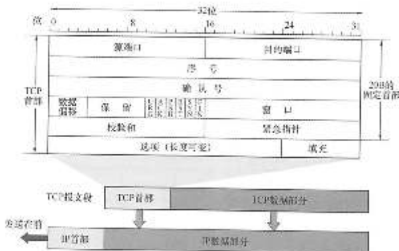
图 5.6 TCP 报文段
