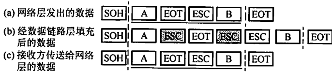
图 3.4 字符填充法
