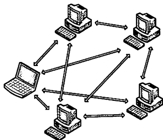
图 6.2 P2P 模型
