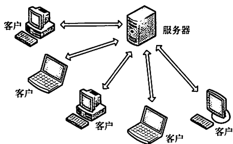
图 6.1 C/S 模型
