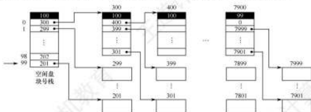
图 4.23 成组链接法示意图
