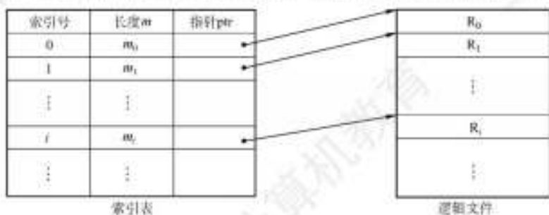
图 4.4 索引文件示意图
