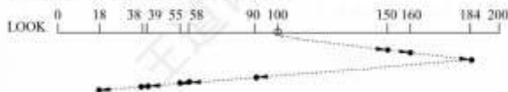
图 5.22 LOOK 磁盘调度算法
