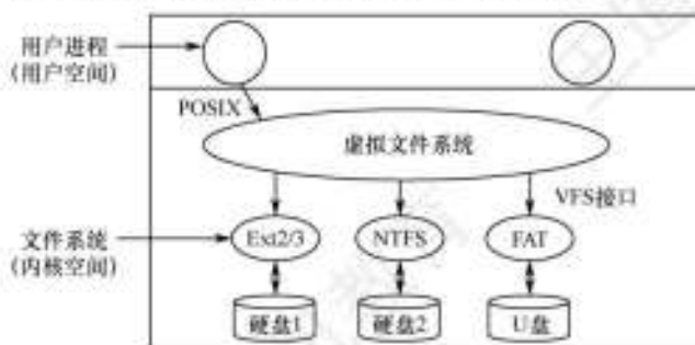
图 4.24 虚拟文件系统的示意图
