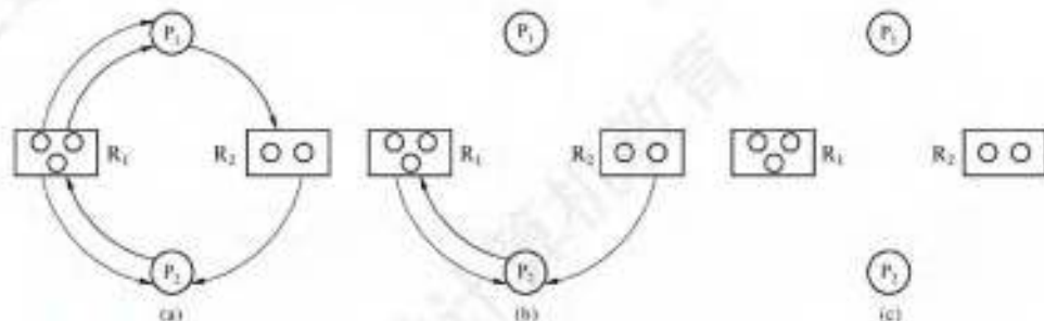
图 2.15 资源分配示例
