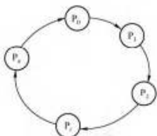
图 2.13 循环等待
