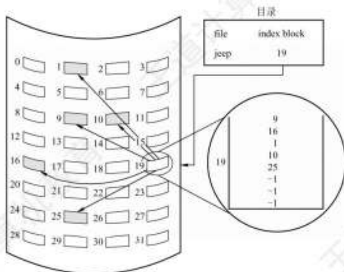
图 4.9 索引分配
