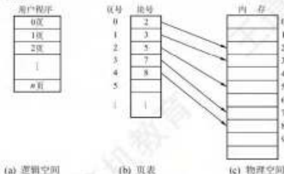
图 3.8 页表的作用
