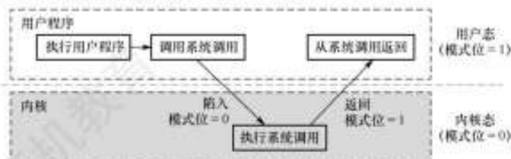
图 1.3 系统调用执行过程
