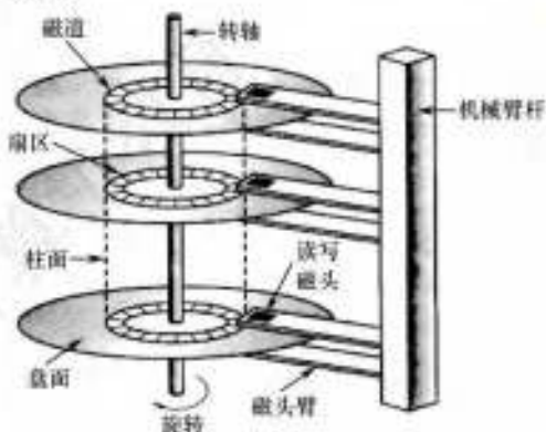
图 5.16 磁盘的结构
