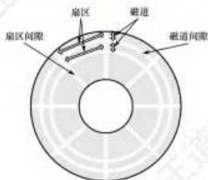
图 5.15 磁盘盘片
