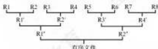
图 8.15 二路平衡归并的排序过程
