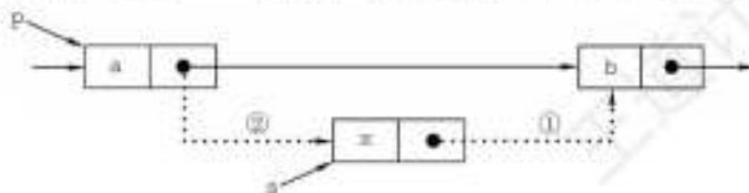
图 2.5 单链表的插入操作
