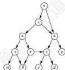
图 6.21 有向无环图描述表达式
