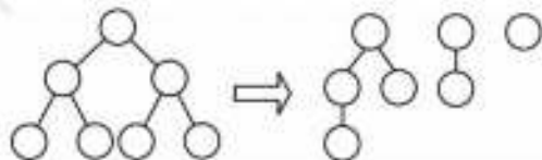
(a) 满二叉树转化为对应的森林
