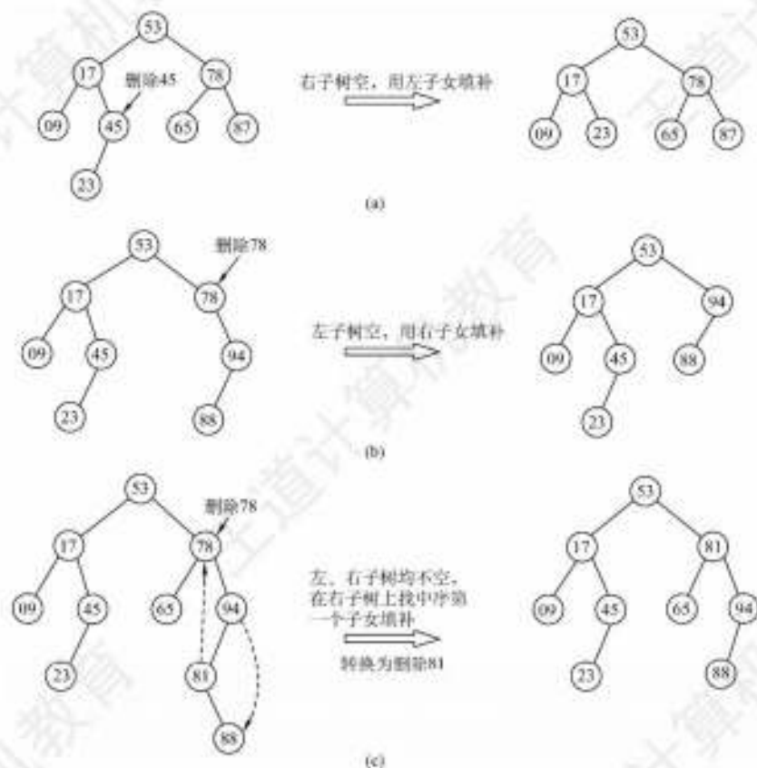
图 7.7 3 种情况下的删除过程
