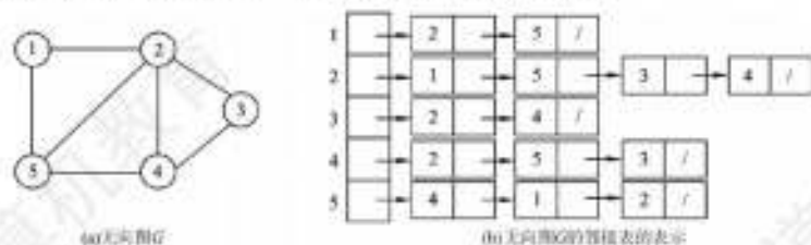
图 6.7 无向图邻接表表示法实例
