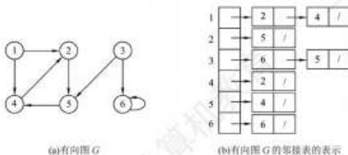
图 6.8 有向图邻接表表示法实例
