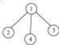
图 6.4 图 G_2 的一个生成树
