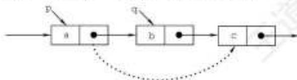
图 2.6 单链表结点的删除
