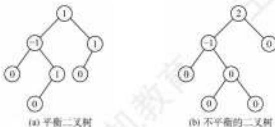
图 7.9 平衡二叉树和不平衡的二叉树
