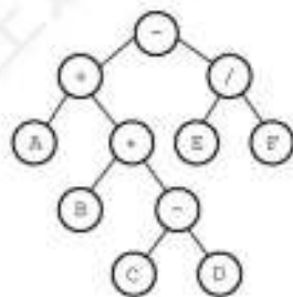
图 3.15 A+B*(C-D)-E/F 对应的表达式树
