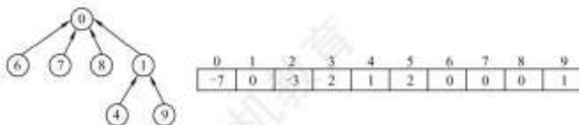
图 5.31 S_1 \cup S_2 可能的表示方法
