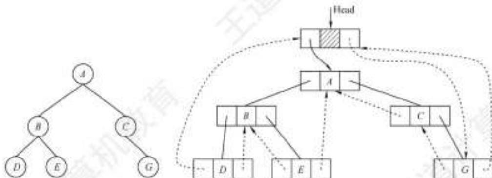
图 5.19 带头结点的中序线索二叉树
