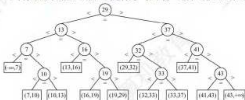
图 7.2 描述折半查找过程的判定树
