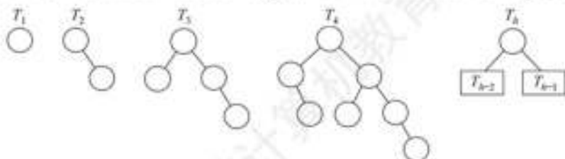
图 7.17 结点数 n 最少的平衡二叉树
