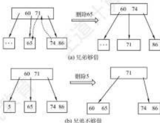
图 7.31 4 阶 B 树中删除终端结点关键字的示意图
