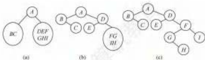
图 5.13 一棵二叉树的构造过程
