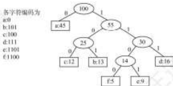
图 5.28 由哈夫曼树构造哈夫曼编码
