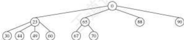
图 1 插入 65 后的树形
