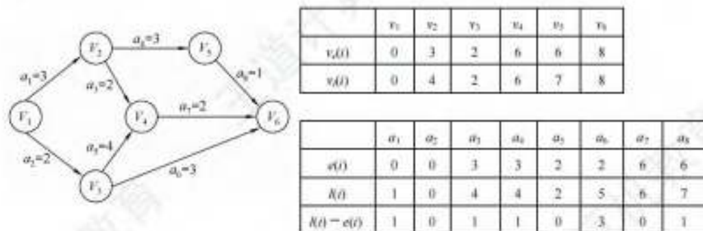
图 6.23 求解关键路径的过程
