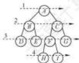
图 5.11 二叉树的层次遍历
