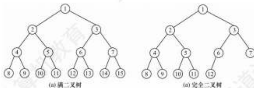
图 5.3 两种特殊形态的二叉树 ①
