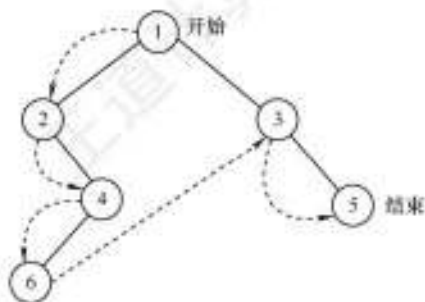
图 5.7 二叉树的先序遍历
