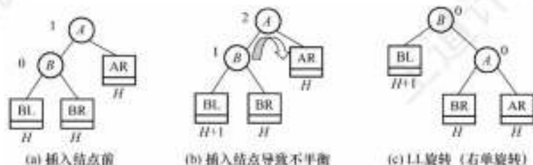
图7.11 LL平衡旋转
