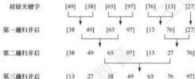
图8.9 二路归并排序示例
