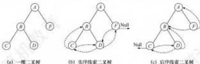
图 5.20 先序线索二叉树和后序线索二叉树
