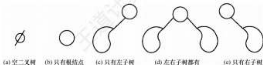
图 5.2 二叉树的 5 种基本形态
