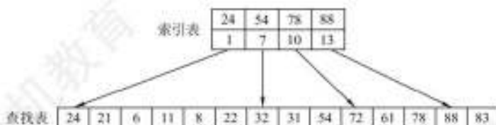
图 7.3 分块查找示意图
