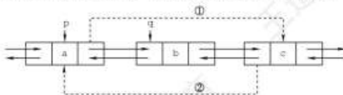
图 2.11 双链表删除结点过程
