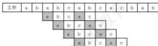
图 4.3 失配后移动情况
