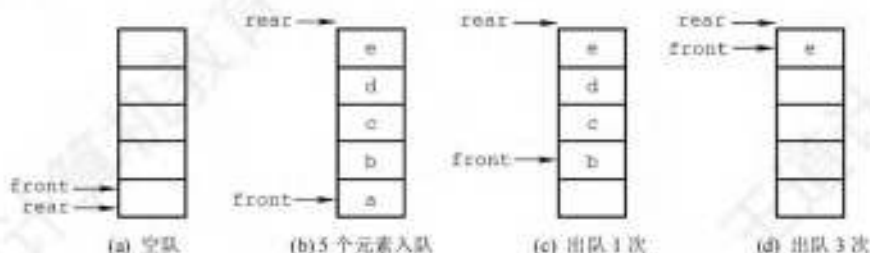
图 3.6 队列的操作
