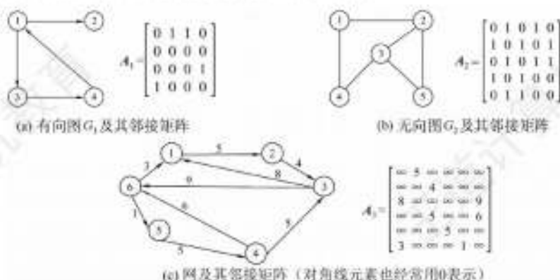
图 6.5 有向图、无向图及网的邻接矩阵
