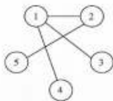
(c) 广度优先生成树
