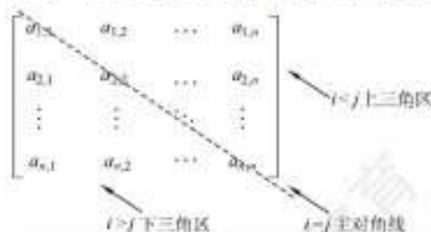
图 3.20 n 阶矩阵的划分
