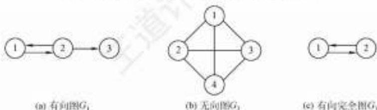
图 6.1 图的示例
