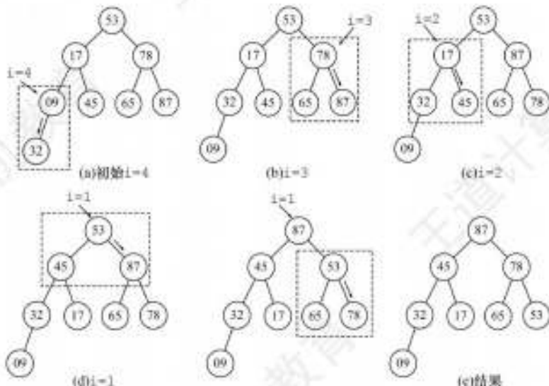
图 8.6 自下往上逐步调整为大根堆
