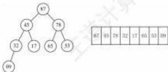
图 8.5 一个大根堆示意图
