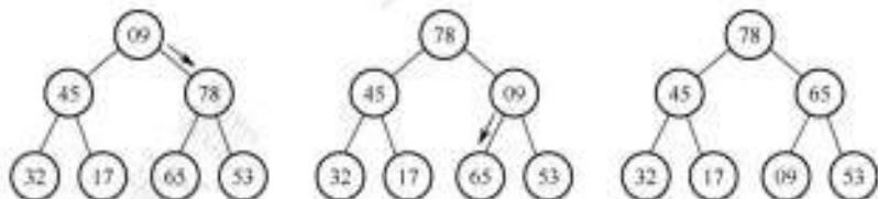
图 8.7 输出堆顶元素后再将剩余元素调整成新堆
