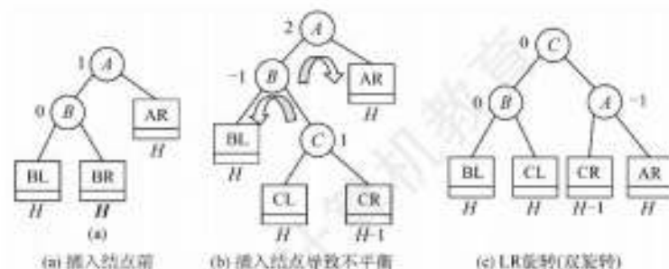
图 7.13 LR 平衡旋转
