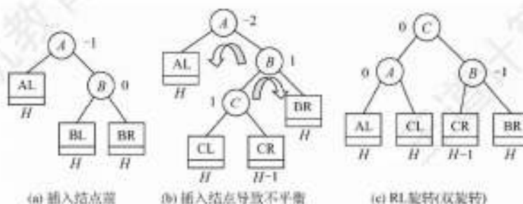
图 7.14 RL 平衡旋转
