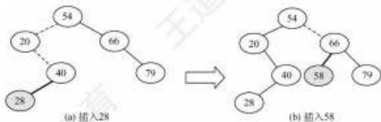
图 7.5 向二叉排序树中插入结点
