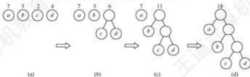
图 5.26 哈夫曼树的构造过程
