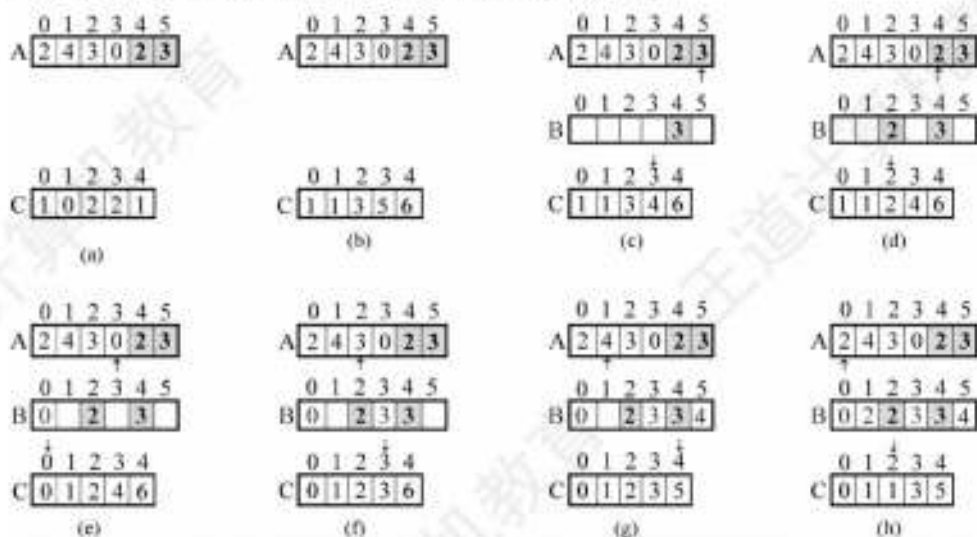
图 8.13 计数排序的过程
