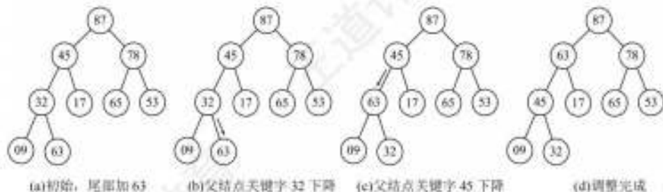
图 8.8 大根堆的插入操作示例
