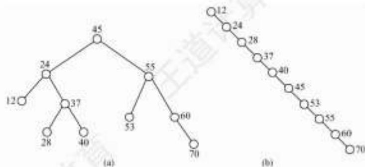
图 7.8 相同关键字组成的不同二叉排序树
