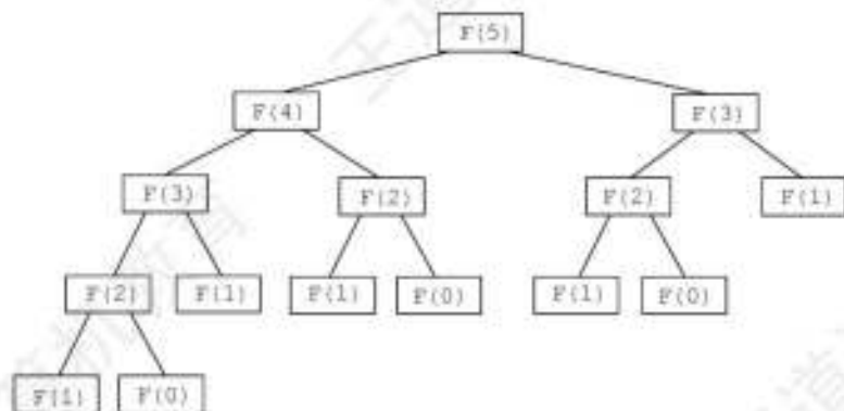
图 3.16 F(5) 的递归执行过程
