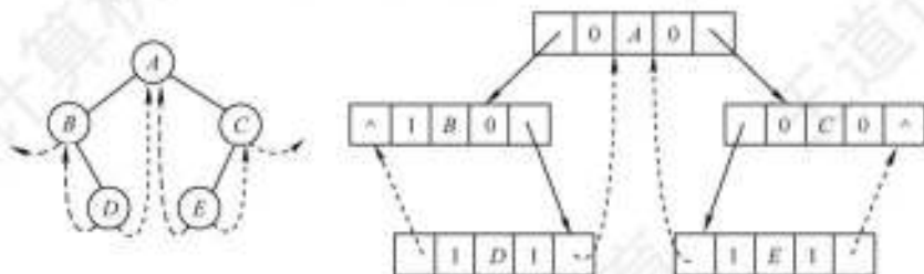
图 5.18 中序线索二叉树及其二叉链表示
