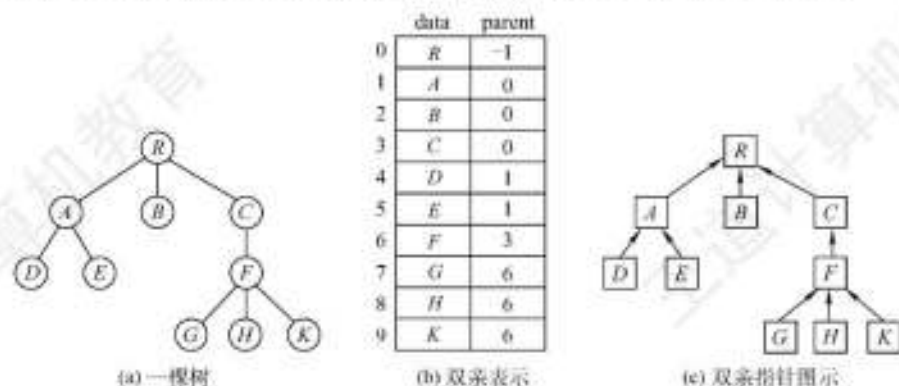
图5.21 树的双亲表示法
