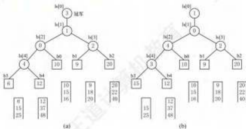
图 8.17 实现 5 路归并的败者树
