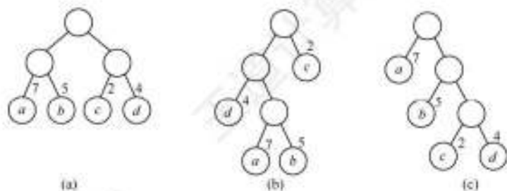
图 5.25 具有不同带权长度的二叉树
