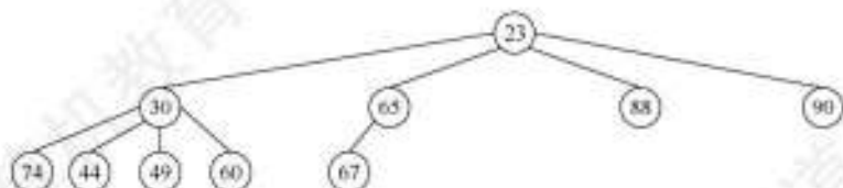
图 2 删除堆顶元素后的树形
