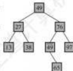
(d) 第四层快排处理后: 最终结果
