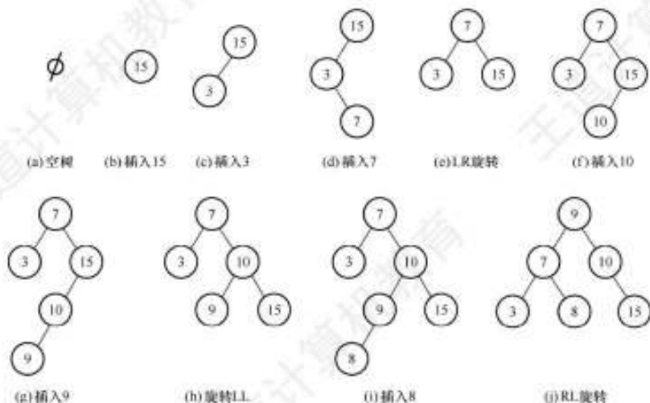
图 7.15 平衡二叉树的生成过程
