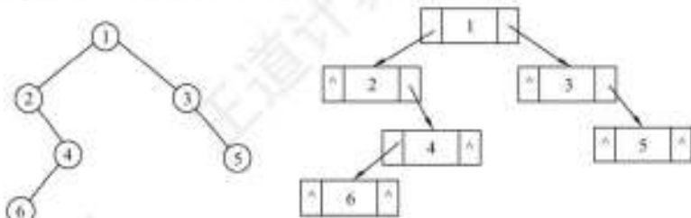
图 5.6 二叉链表的存储结构
