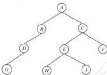
图 3.17 二叉树
