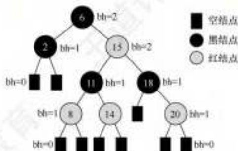
图 7.18 一棵红黑树
