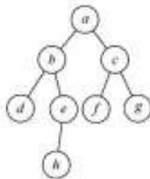
图 6.11 一个无向图 G
