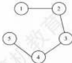
(b) 深度优先生成树
