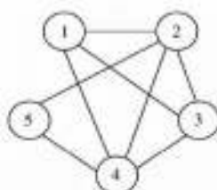
(a) 图G
