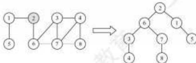
图 6.12 图的广度优先生成树
