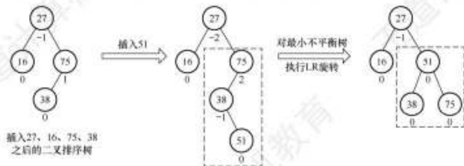
图7.10 最小不平衡子树示意
