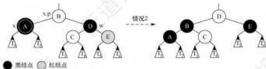
图 7.24 情况 2 的调整方式
