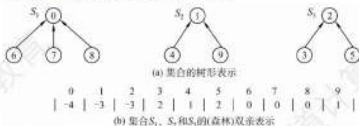
图 5.30 用树表示并查集
