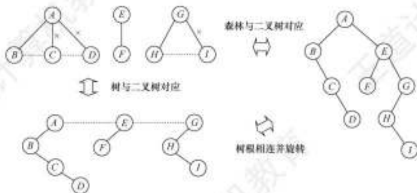
图 5.24 森林与二叉树的对应关系
