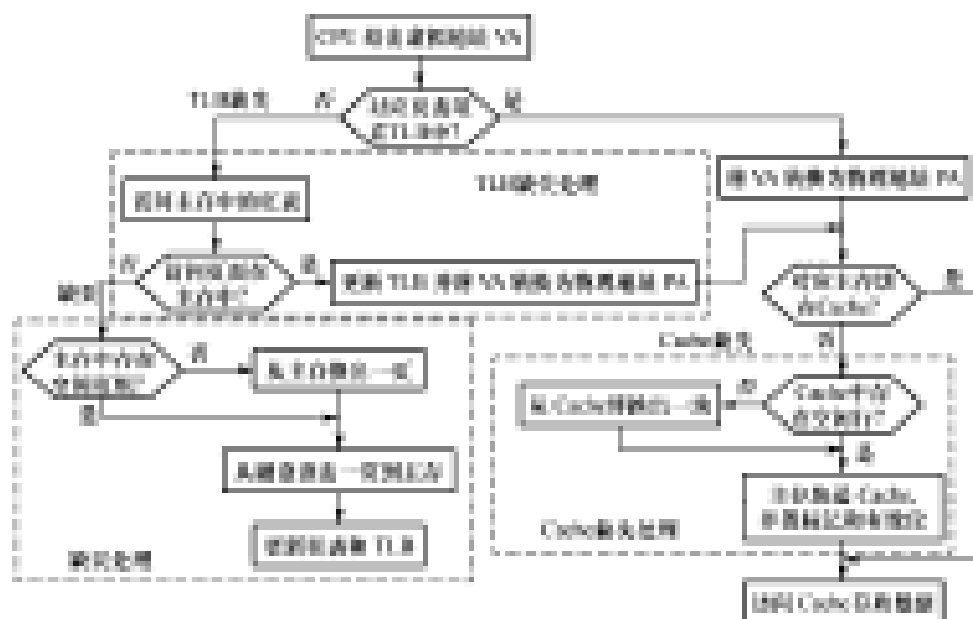
图 3.30 带 TLB 虚拟存储器的 CPU 访存过程
