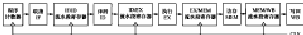
图 5.17 流水线的逻辑结构图
